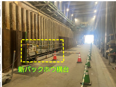
新構台設置&旧基礎撤去の完了状況
