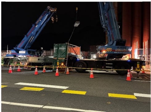
型枠設置作業状況（夜間）
