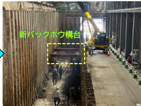
土砂ピット上にバックホウ構台設置
