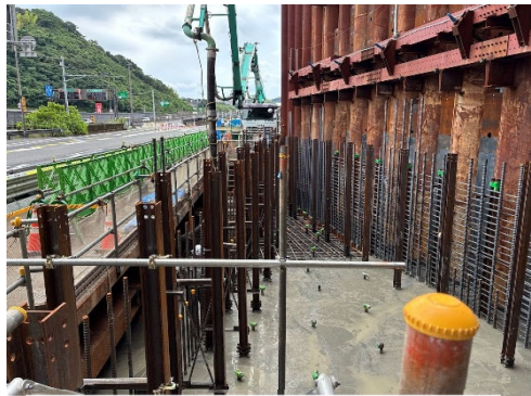
コンクリート打設作業状況 ※擁壁のフーチング（土台）が完了し壁部の作業を行っています
