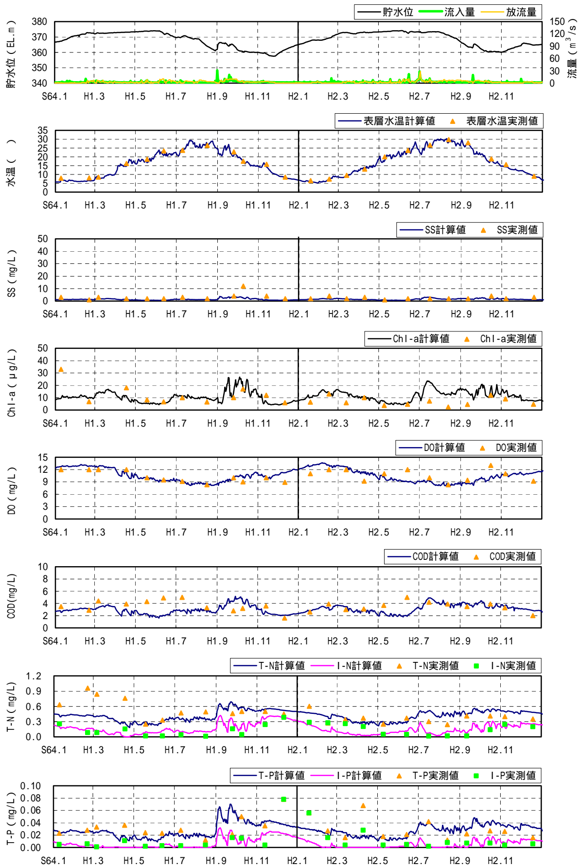
図 4.1.4.2-13 水質の検証結果(北山ダム貯水池地点表層)(1/5)
