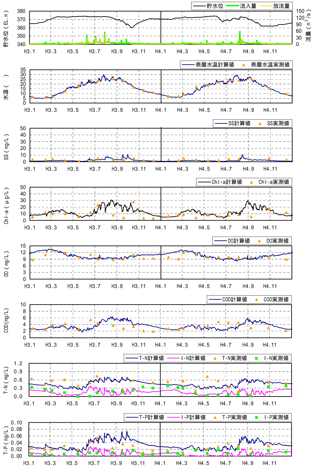
図 4.1.4.2-13 水質の検証結果(北山ダム貯水池地点表層)(2/5)
