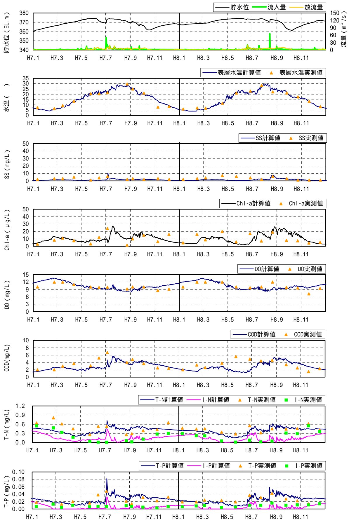
図 4.1.4.2-13 水質の検証結果(北山ダム貯水池地点表層)(4/5)
