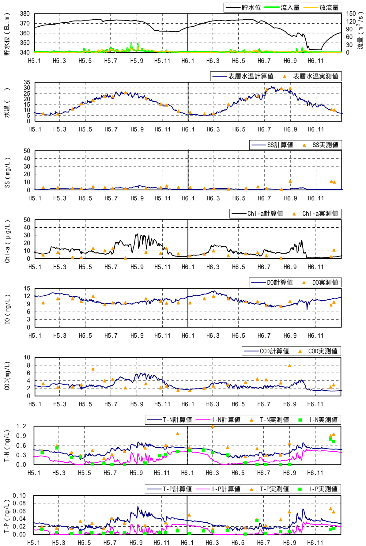
図 4.1.4.2-13 水質の検証結果(北山ダム貯水池地点表層)(3/5)
