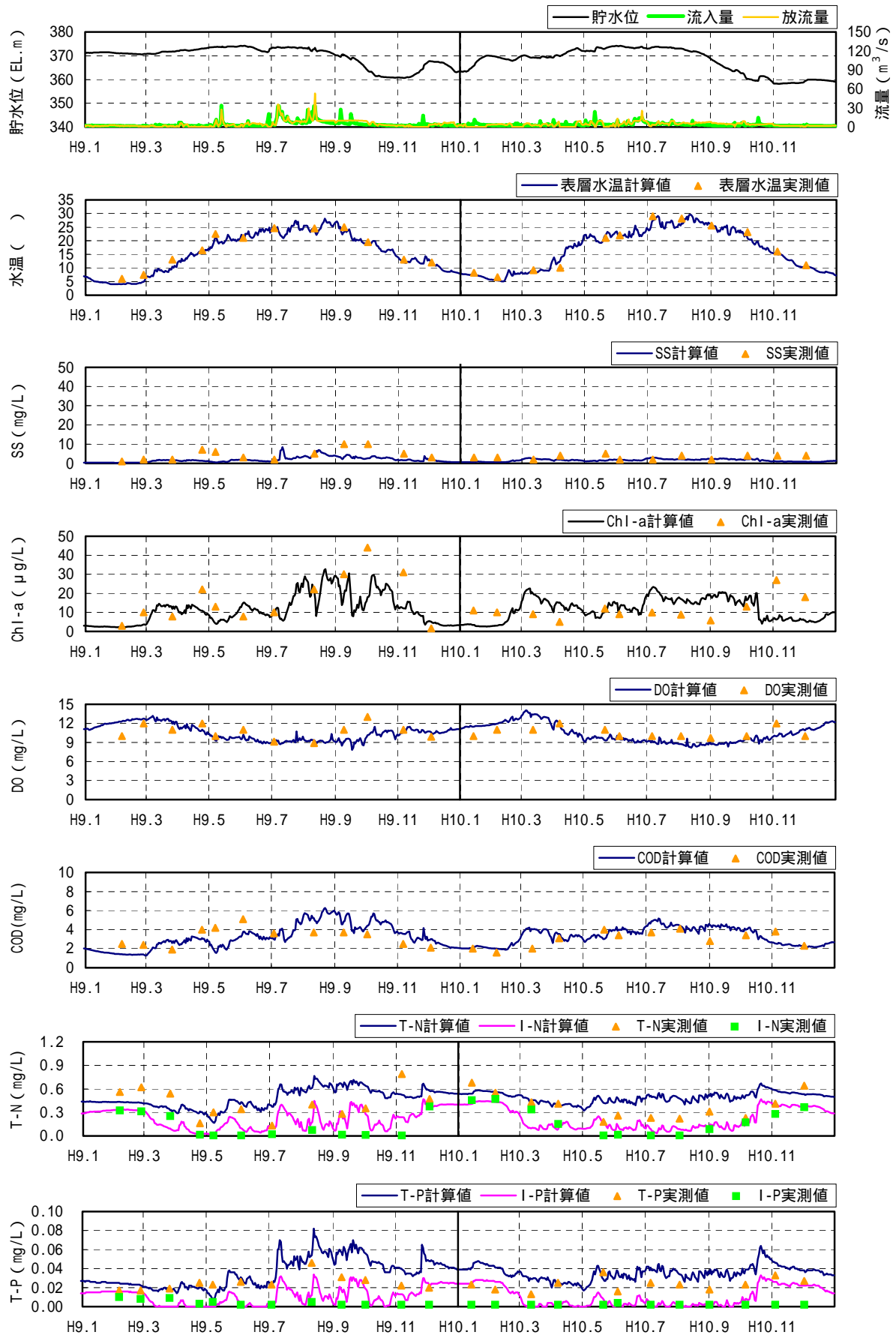
図 4.1.4.2-13 水質の検証結果(北山ダム貯水池地点表層)(5/5)
