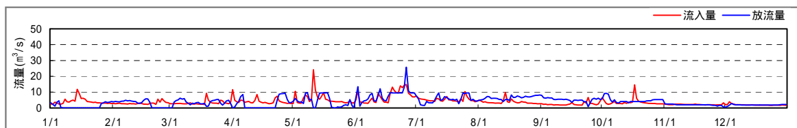
図 4.1.4.2-23(3) T-N 及び T-P の検証結果(北山ダム貯水池地点鉛直分布、平成 10 年)
