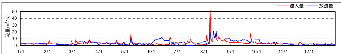
図 4.1.4.2-17(2) DO 及び COD の検証結果(北山ダム貯水池地点鉛直分布、平成 4 年)
