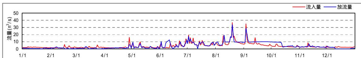
図 4.1.4.2-18(3) T-N 及び T-P の検証結果(北山ダム貯水池地点鉛直分布、平成 5 年)
