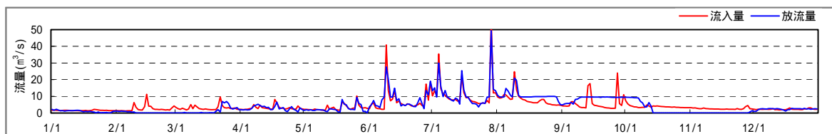
図 4.1.4.2-16(1) 水温及び SS の検証結果(北山ダム貯水池地点鉛直分布、平成 3 年)
