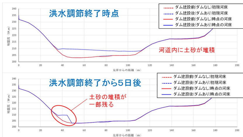
令和2年洪水による堆積箇所(川辺川 22.0k 地点)
