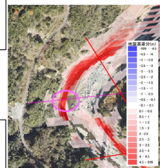
洪水調節終了から5日後の堆積状況
