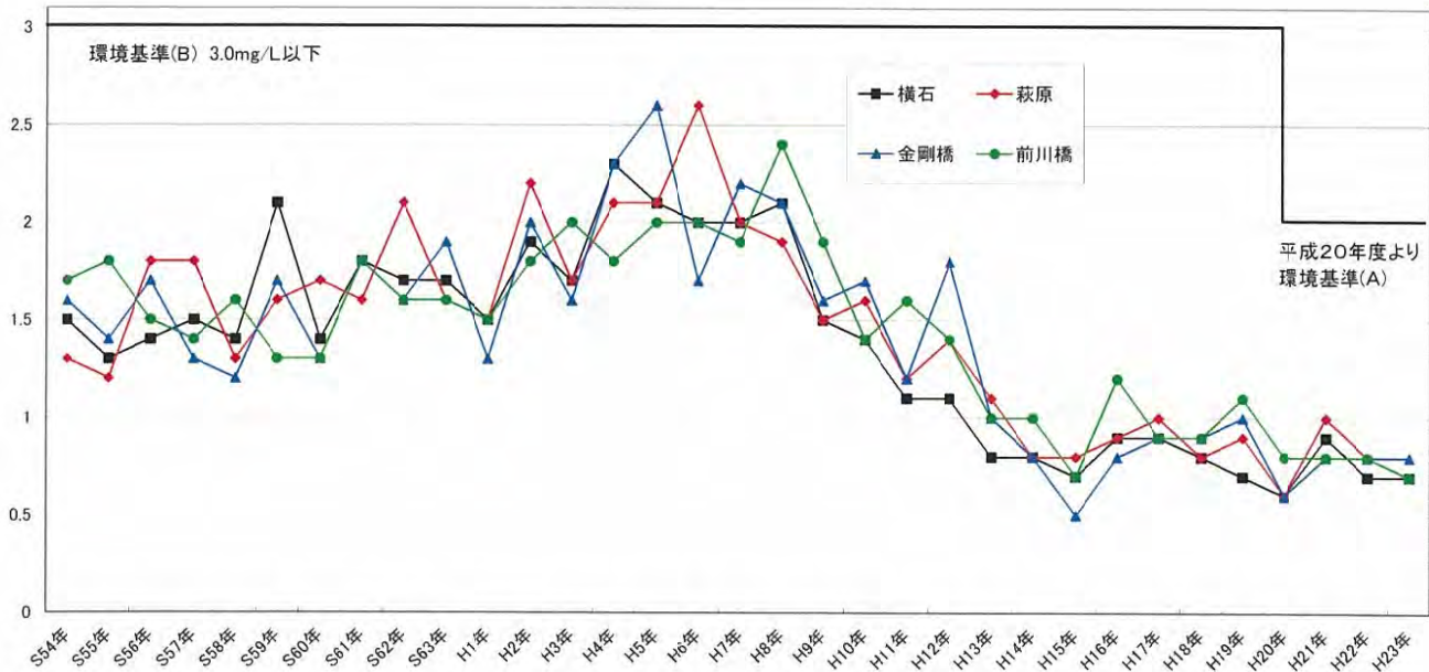
球磨川下流域における水質変化 水質経年変化図 (BOD75%値)
