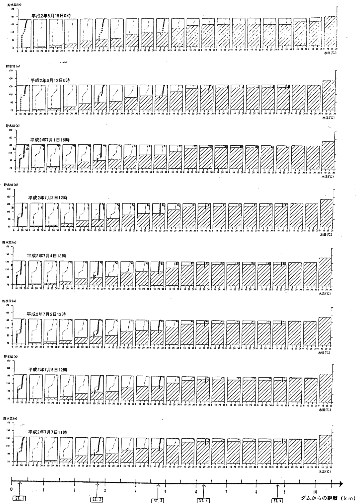
付図 4.2-1 (2) 水質予測モデルの検証計算結果 (水温鉛直分布)
