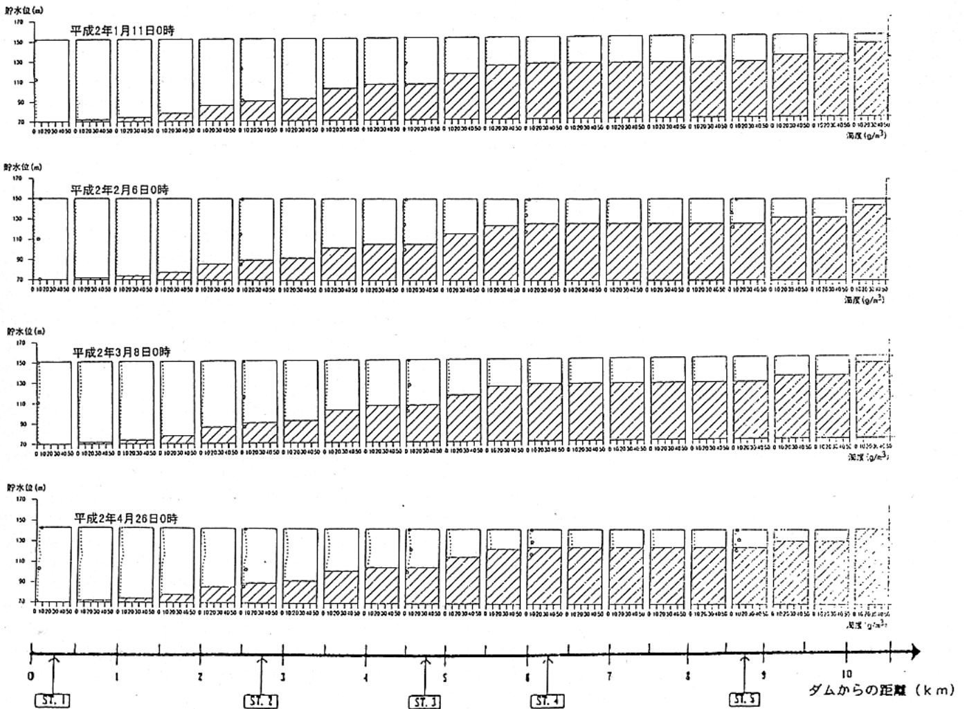
付図 4.2-2 (1) 水質予測モデルの検証計算結果 (濁度鉛直分布)
