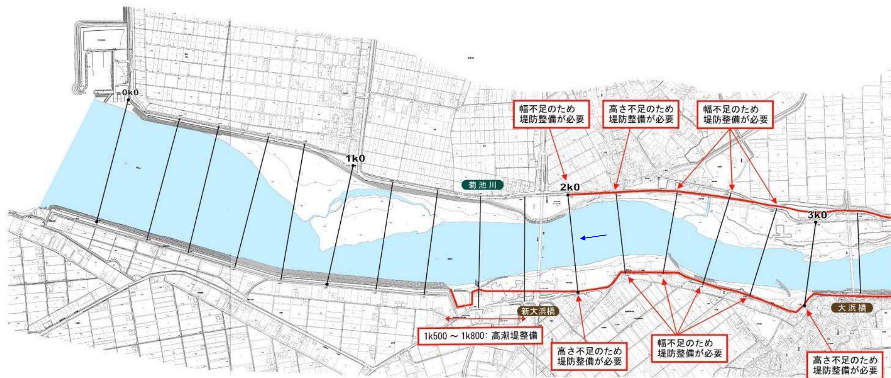
附図1-1 洪水対策に関する施工の場所(国土交通省) (菊池川 河口～3k200)
