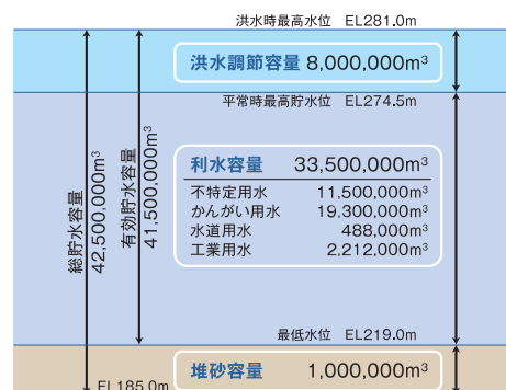
貯水容量分配図
