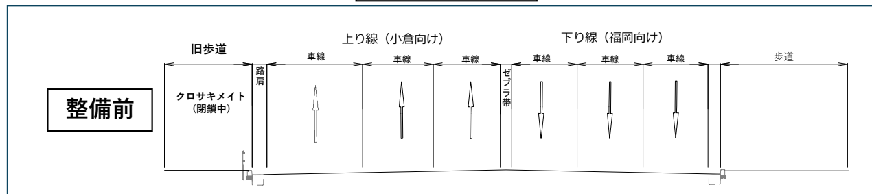
A-A' 断面
