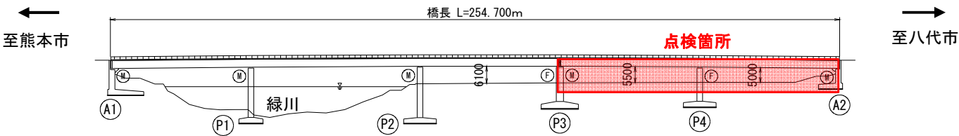
側面図
