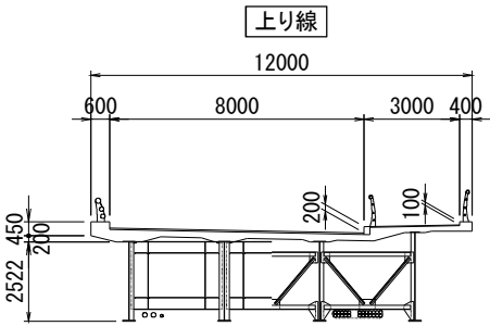
標準断面図
