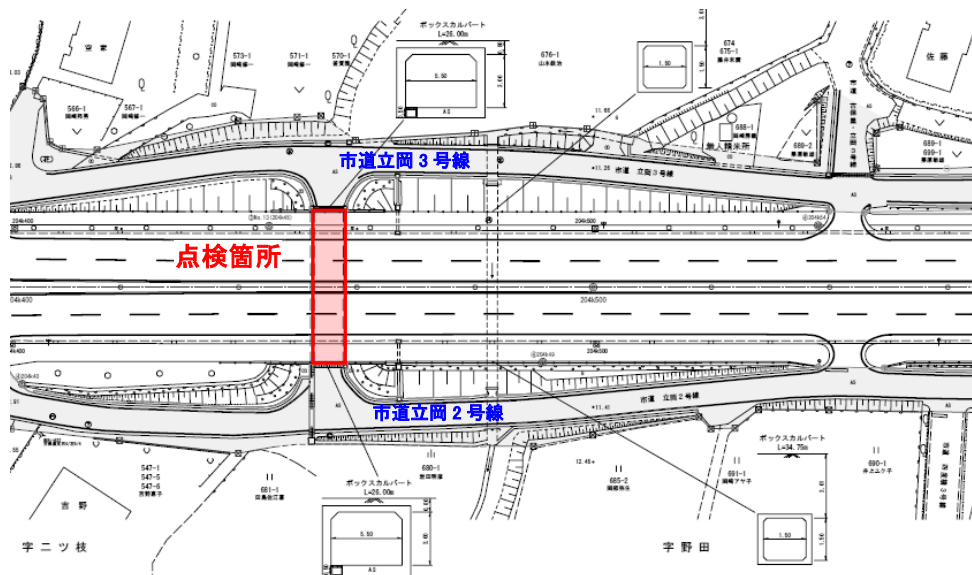
平面図
