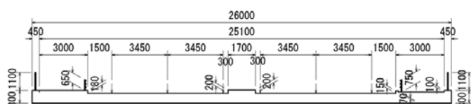
標準断面図
