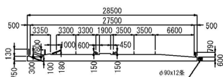
標準断面図
