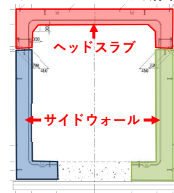
ボックスカルバート断面図
