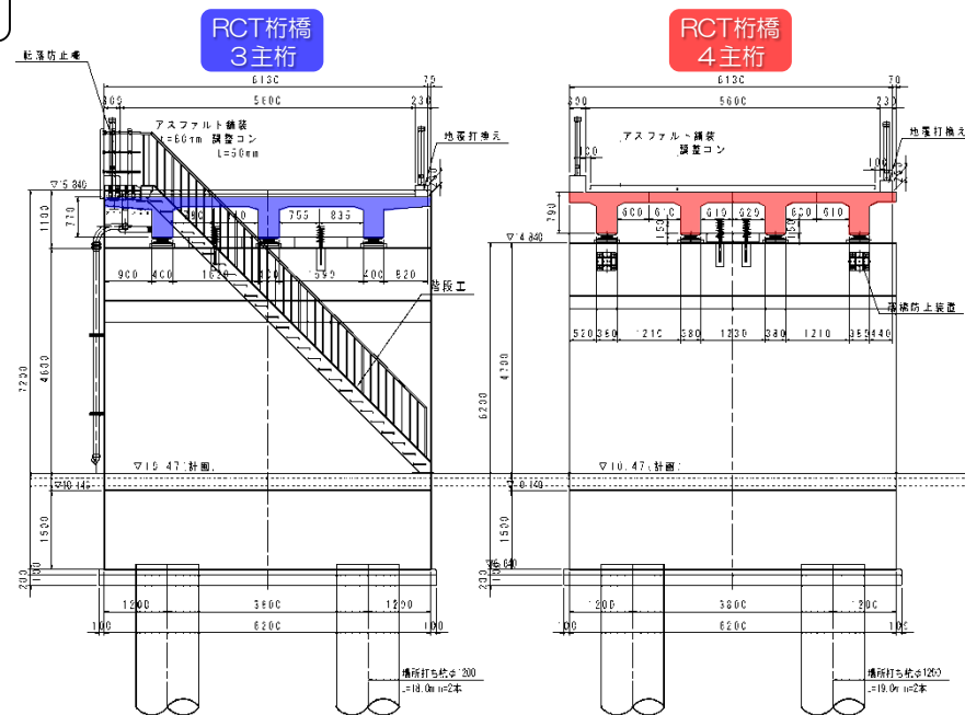
断面図
