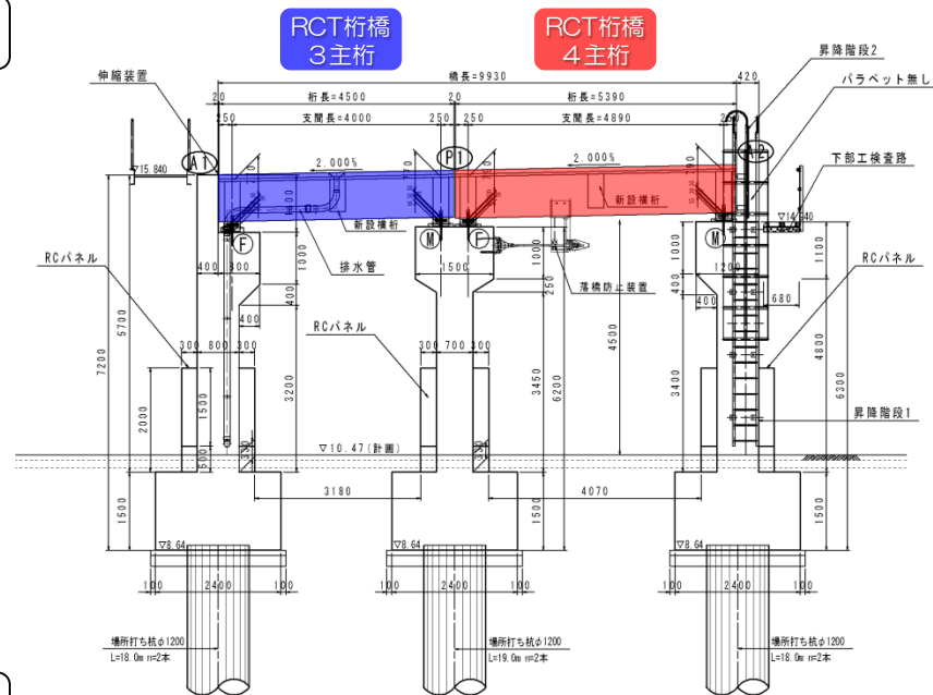
側面図
