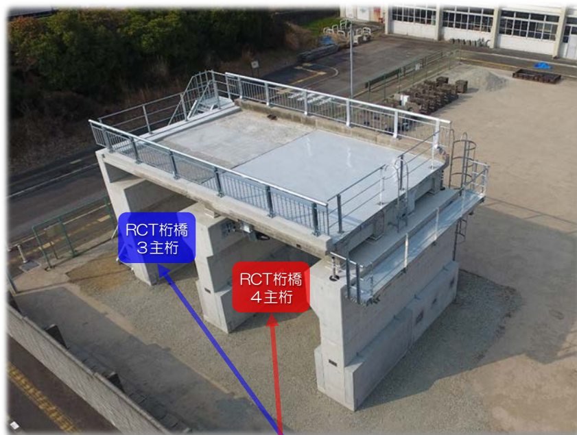
全体図
