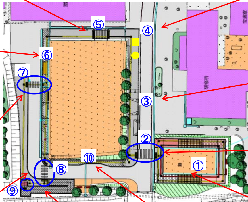
⑨ スロープ体験 縦断勾配(5%)
