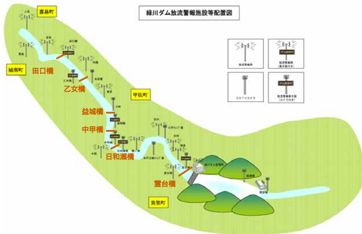
緑川ダム放流警報施設配置図
