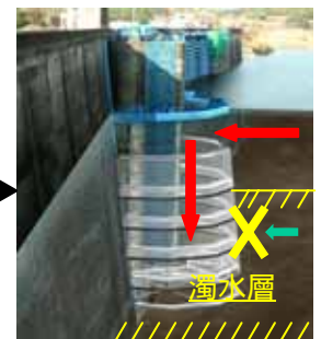
選択取水設備使用時
