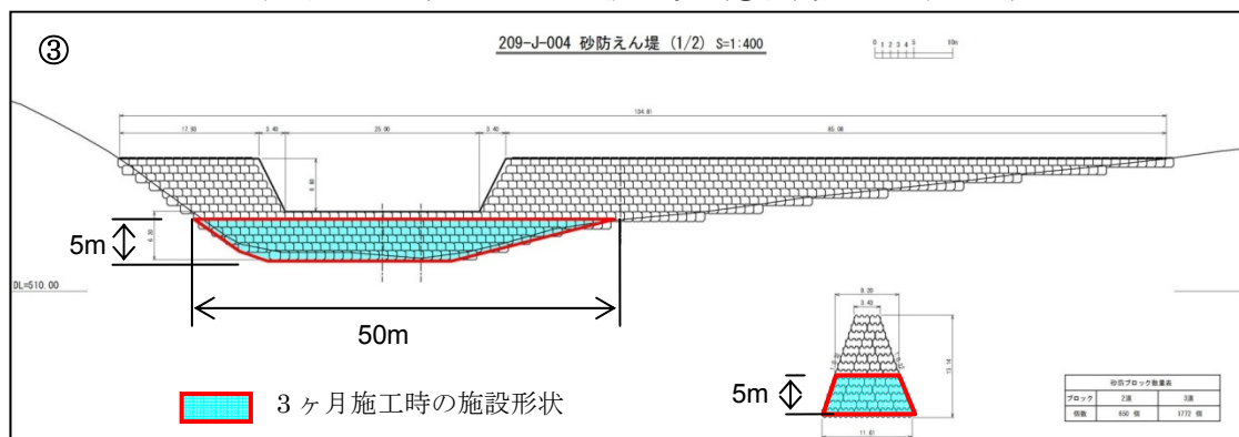
施工開始から 3 ヶ月時点の施設形状 (③出水川応急堰堤工)
