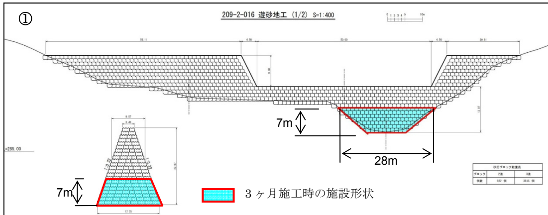
施工開始から 3 ヶ月時点の施設形状 (①白鳥川応急遊砂地工)
