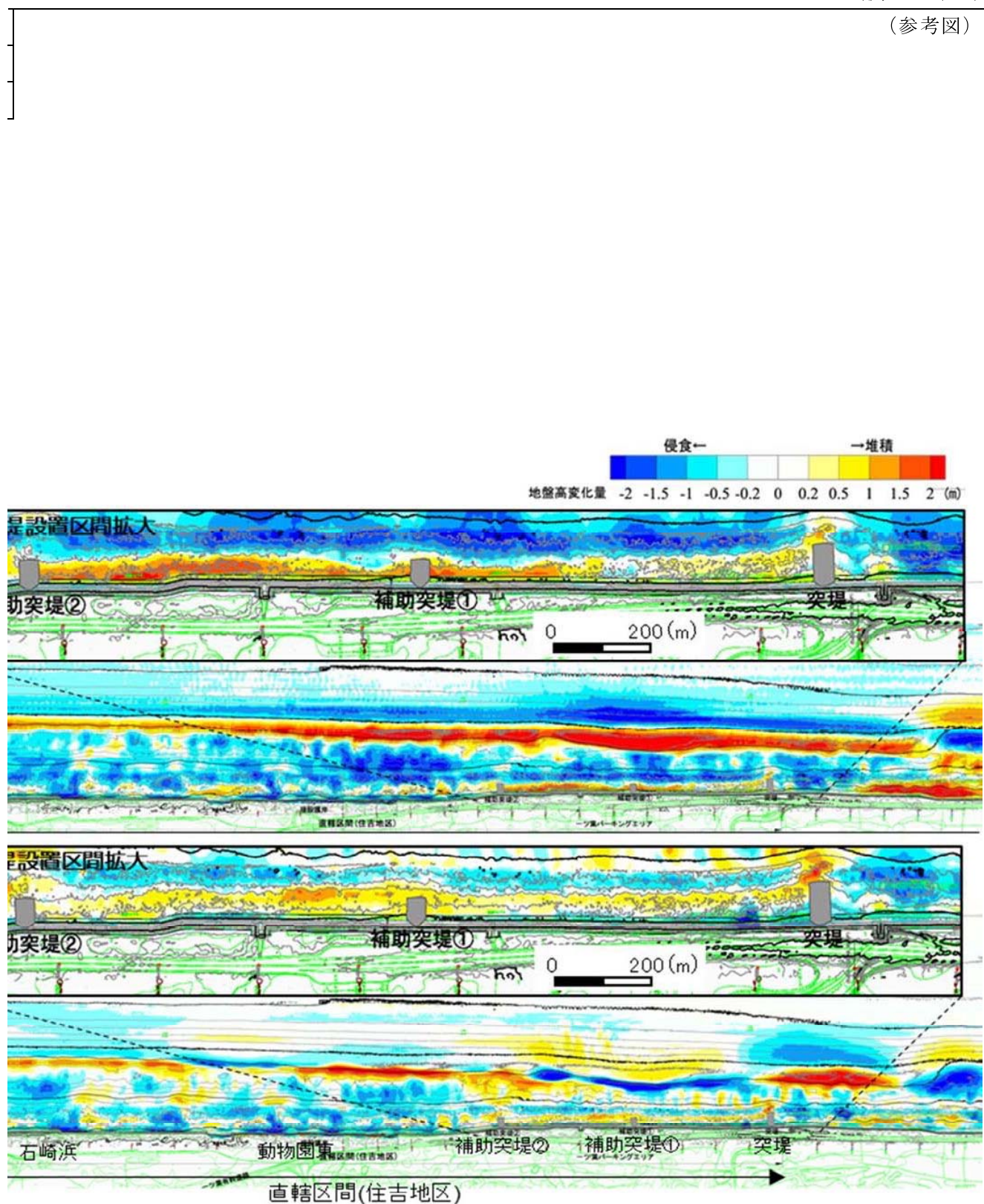
図 宮崎海岸の地盤高変化量の平面分布図
