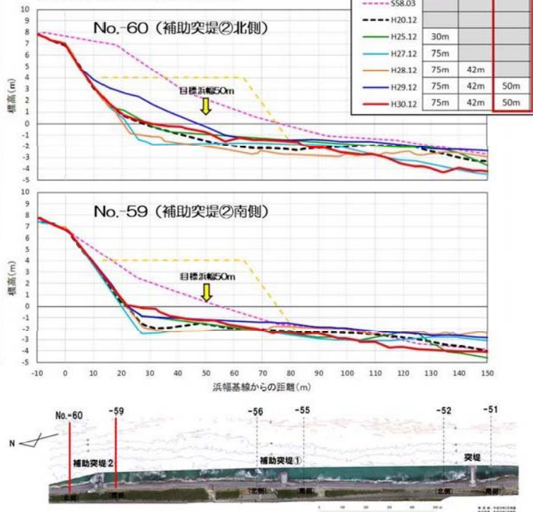
図 補助突堤②周辺の断面変化状況（詳細）
