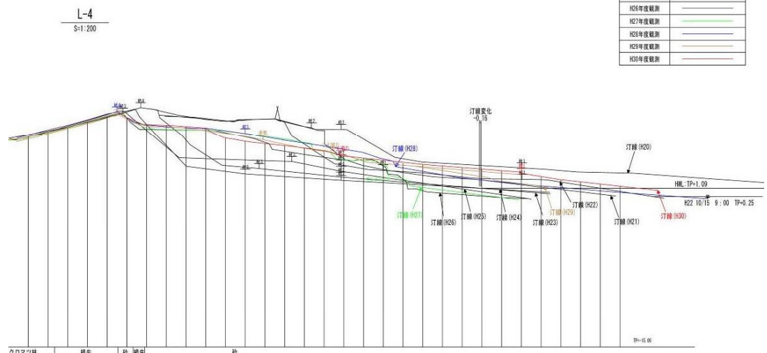
地形の経年変化（簡易横断測量結果重ね図）
