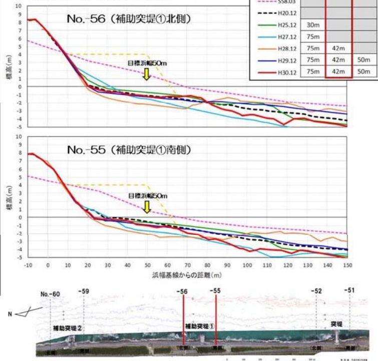
図 補助突堤①周辺の断面変化状況（詳細）
