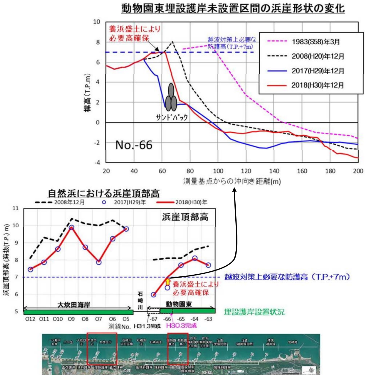
図 動物園東埋設護岸未設置区間の浜崖形状の変化
