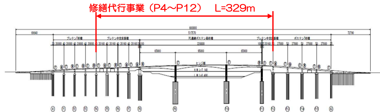
側面図
