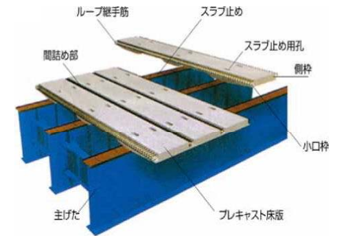
プレキャスト床版
