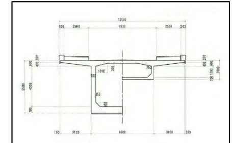
標準断面図
