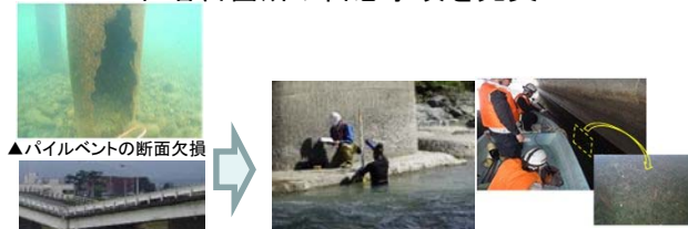
▲潜水士による洗掘調査
