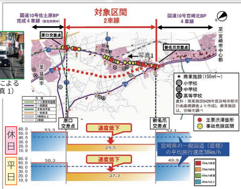
▲国道 10 号対象区間の速度分布図 (ピーク時間帯上下平均)
