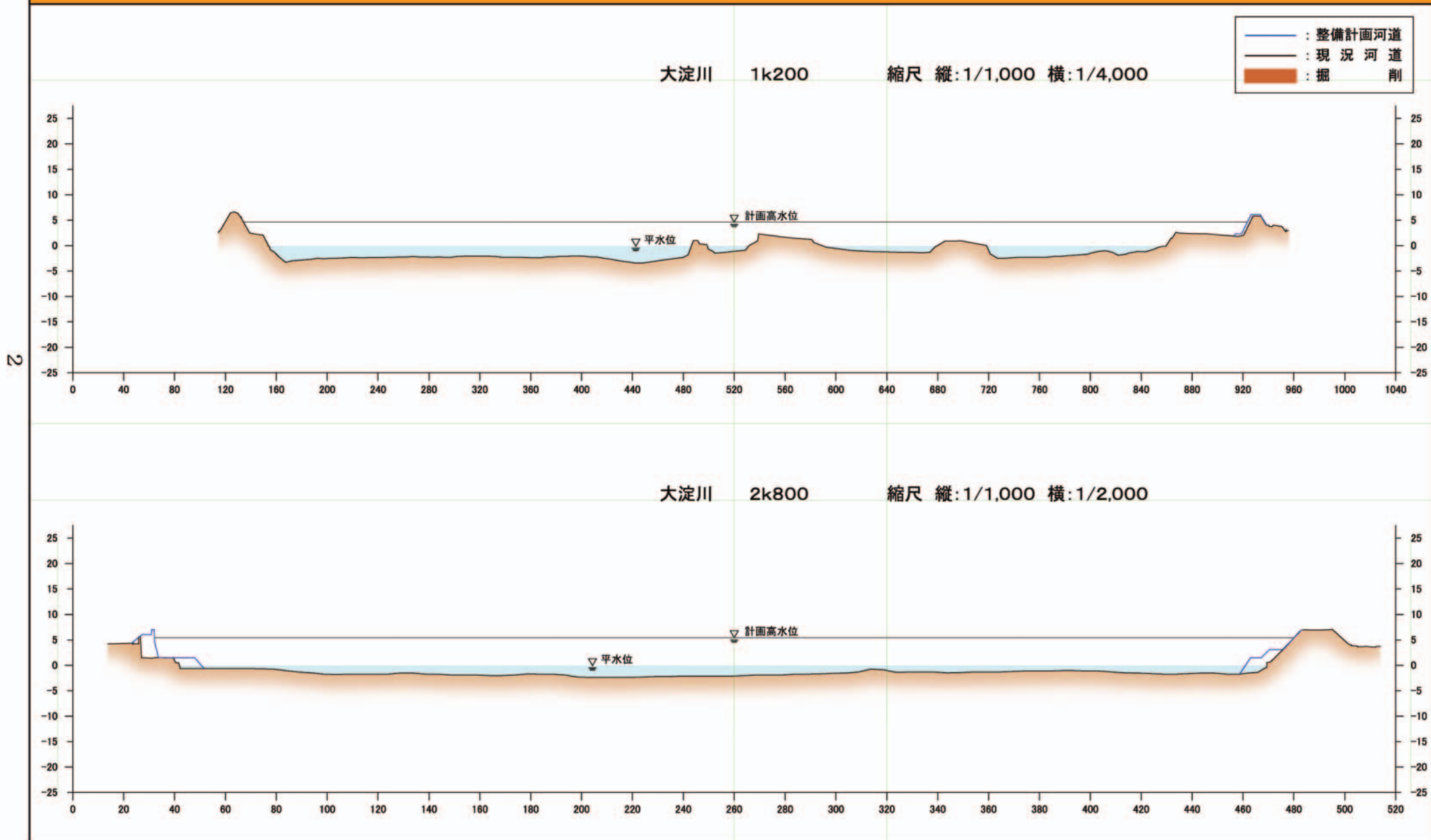
附図2 大淀川横断図(国土交通省)
