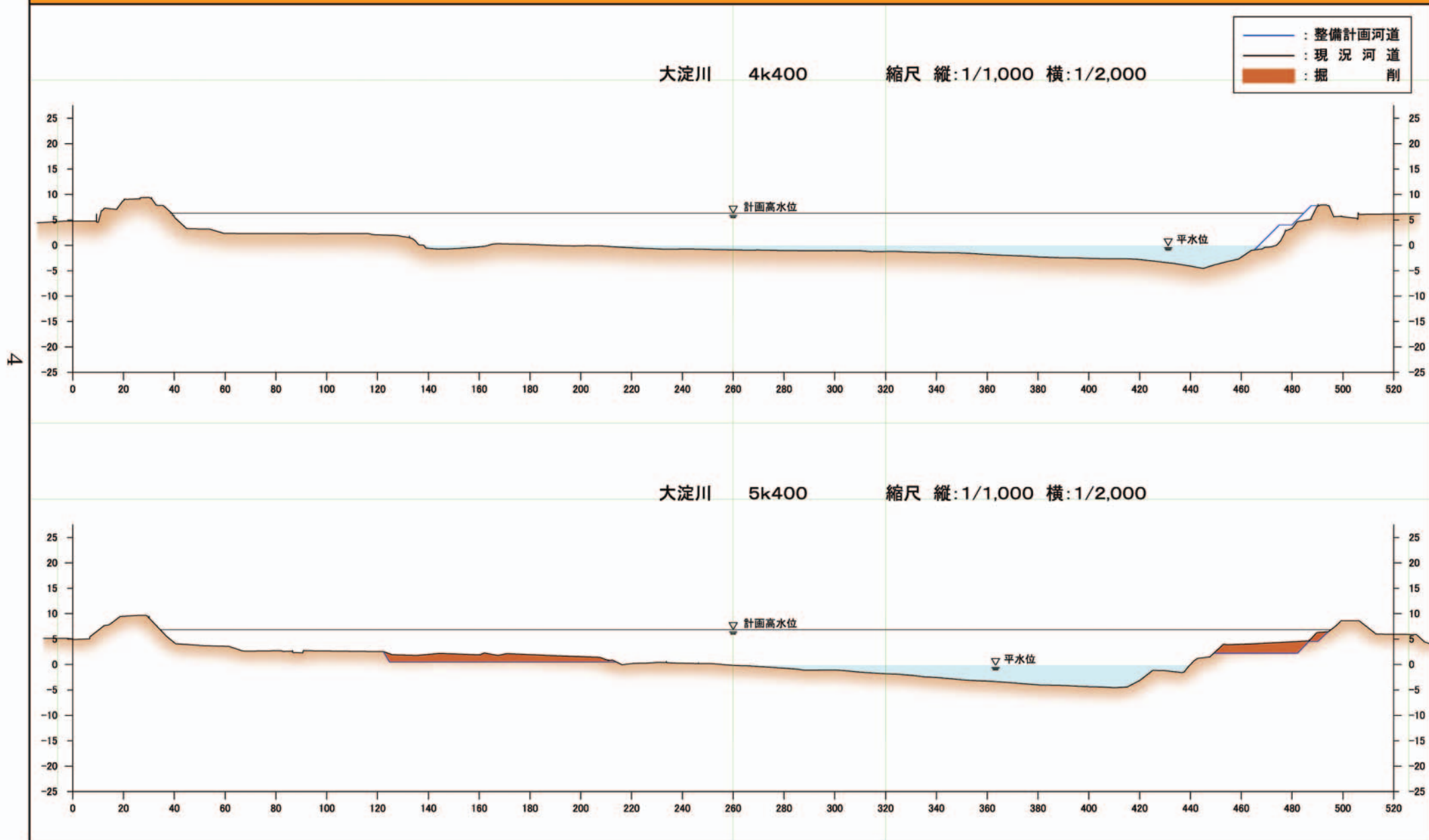
附図4 大淀川横断図(国土交通省)
