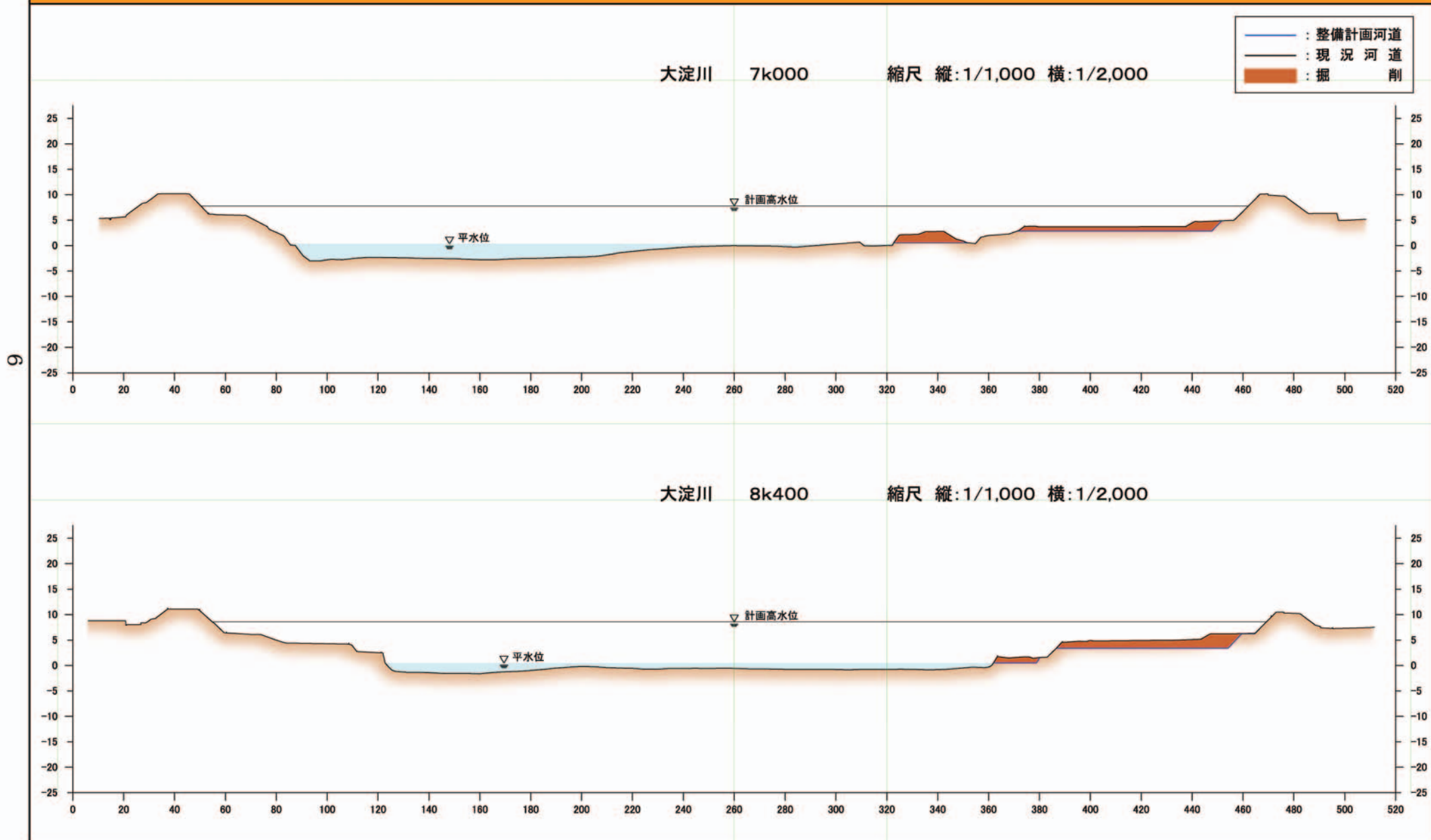
附図6 大淀川横断図(国土交通省)
