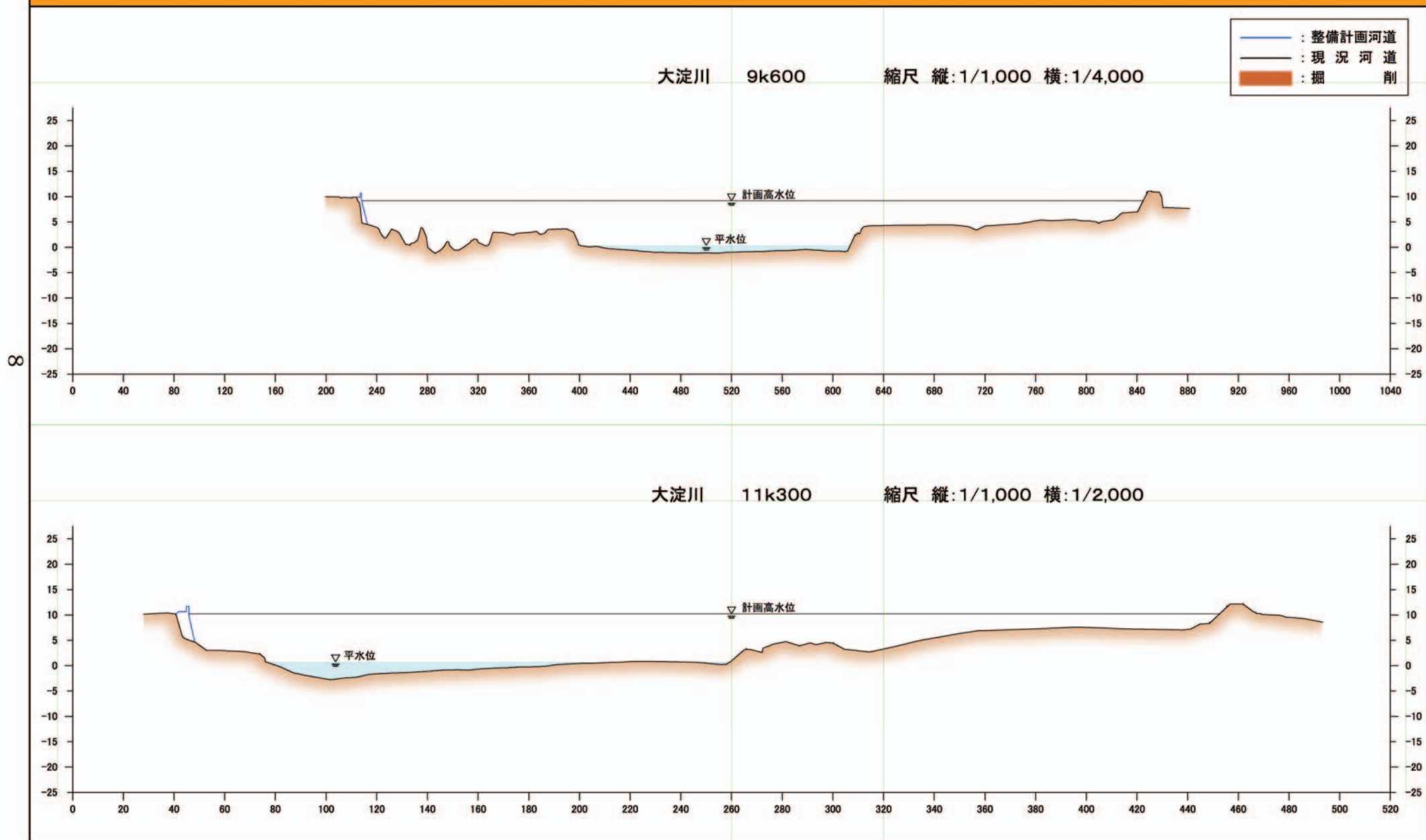
附図8 大淀川横断図(国土交通省)
