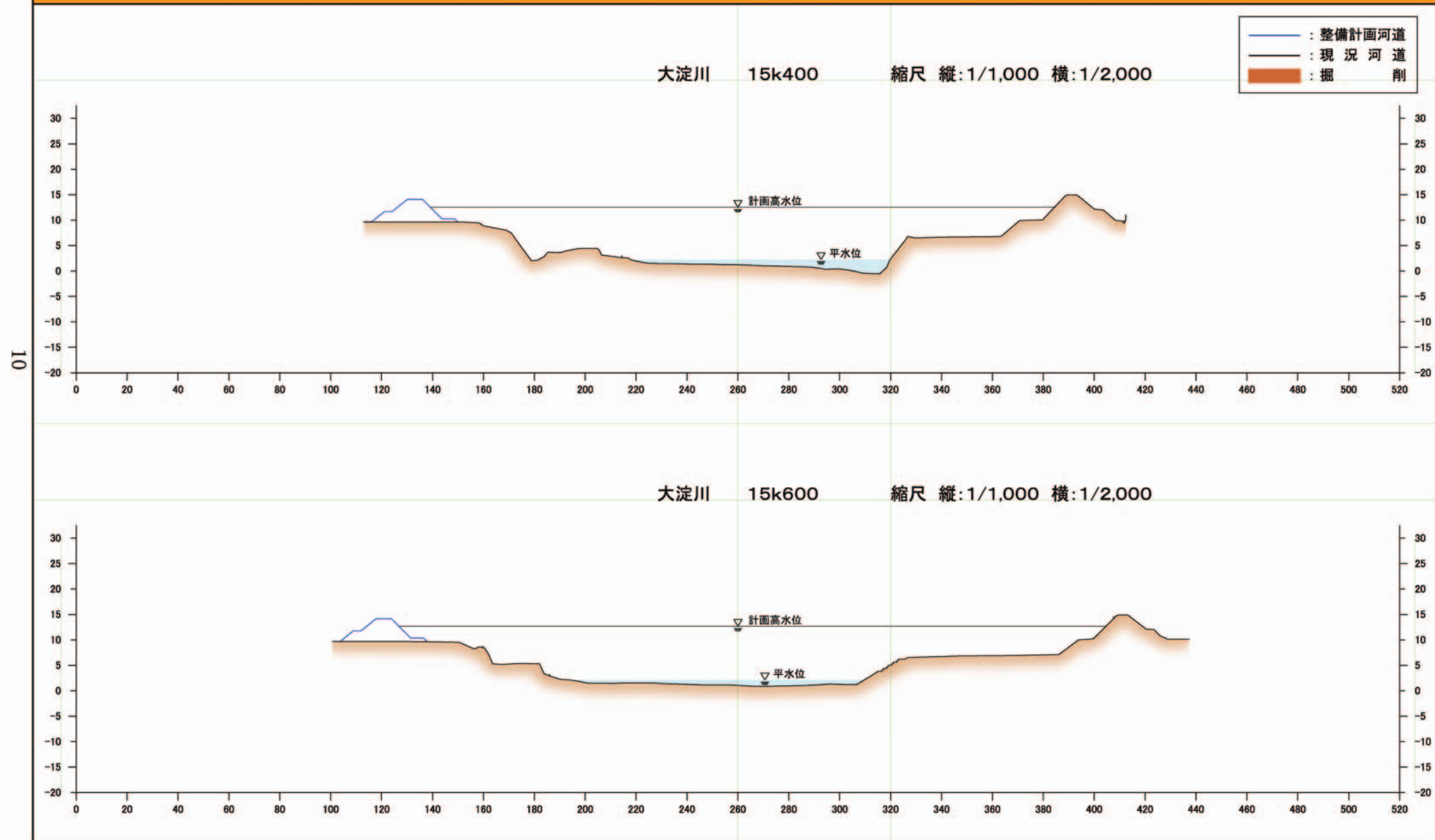
附図10 大淀川横断図(国土交通省)
