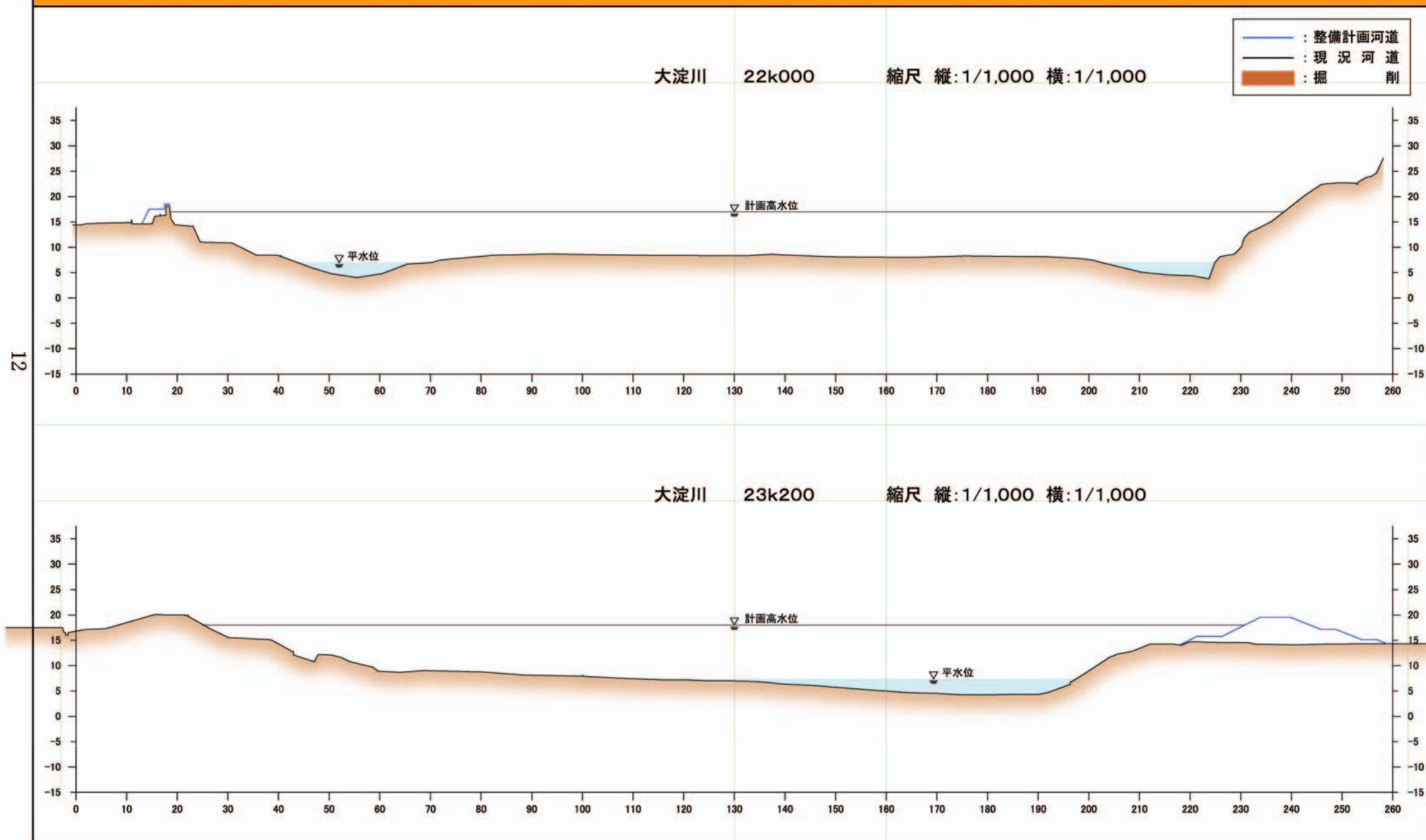
附図12 大淀川横断図(国土交通省)
