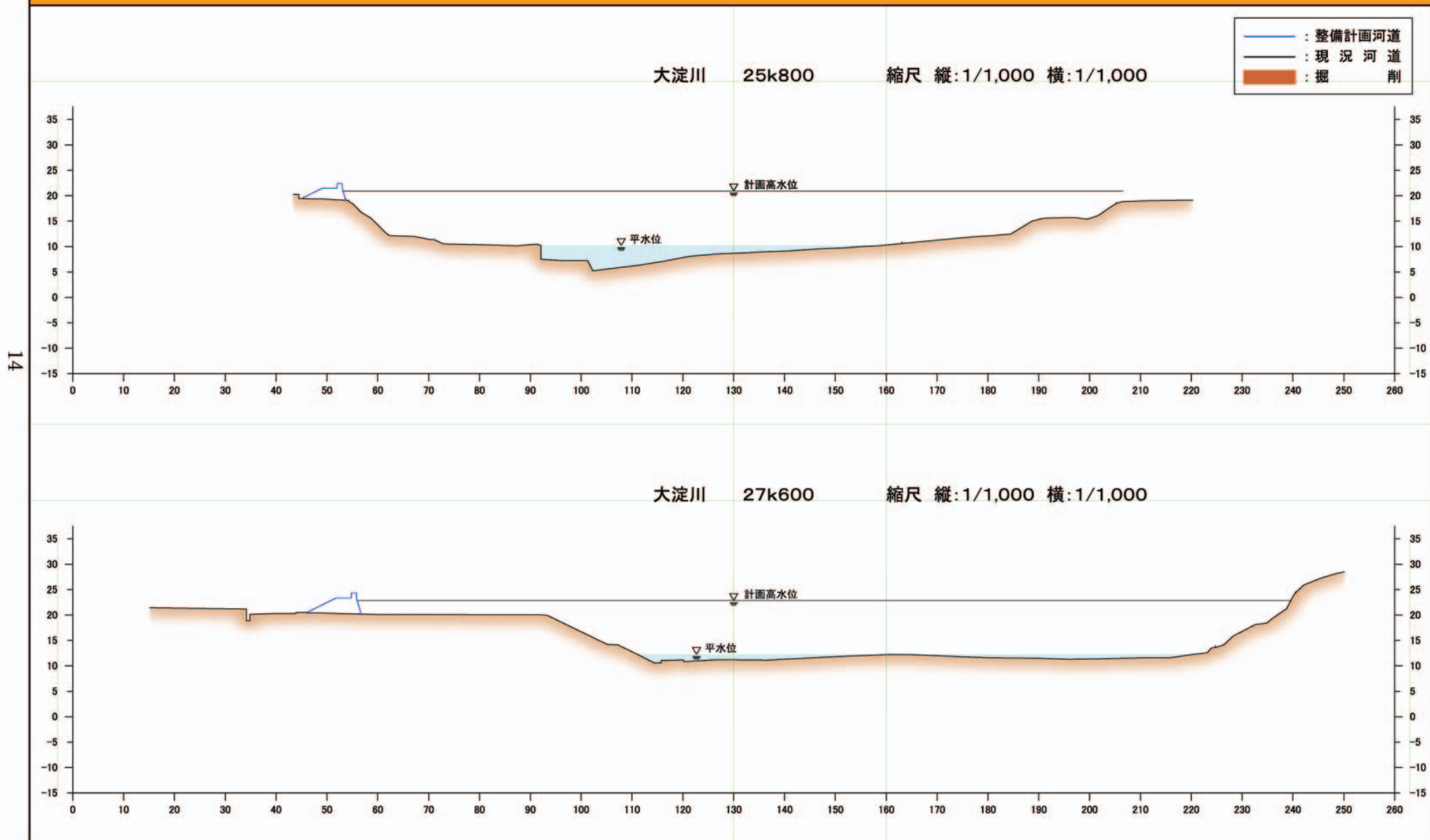
附図14 大淀川横断図(国土交通省)
