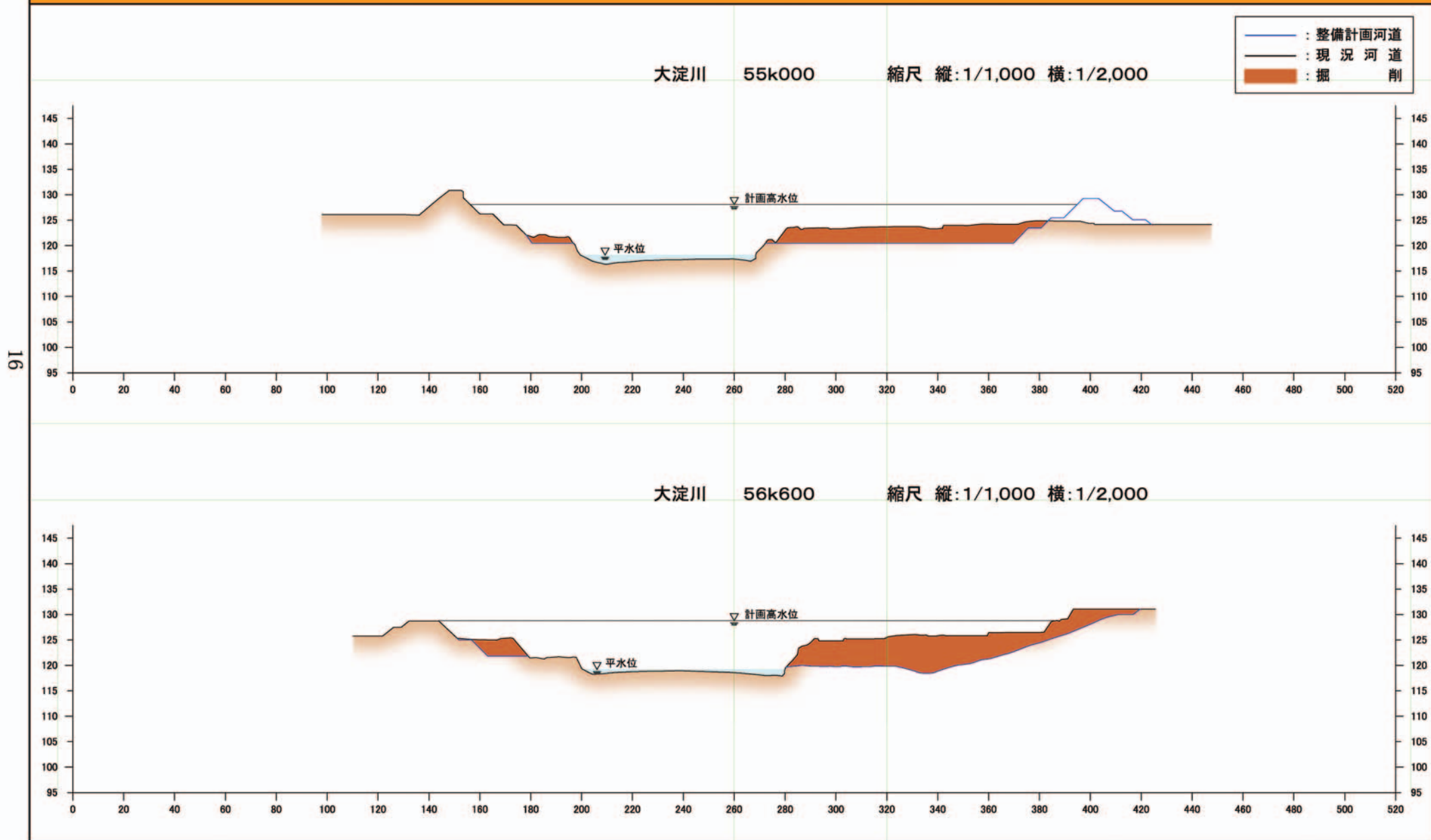
附図16 大淀川横断図(国土交通省)
