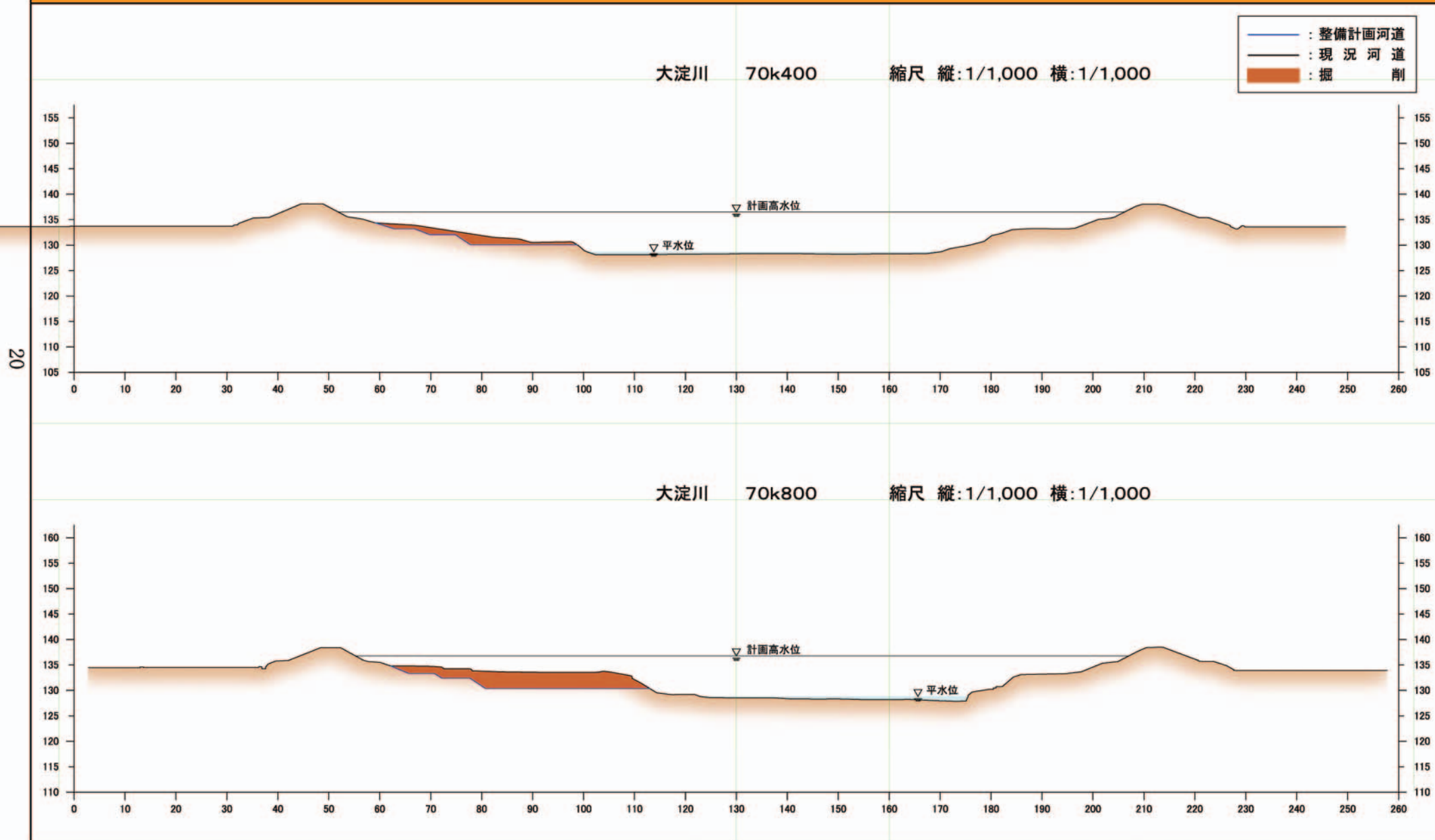
附図20 大淀川横断図(国土交通省)
