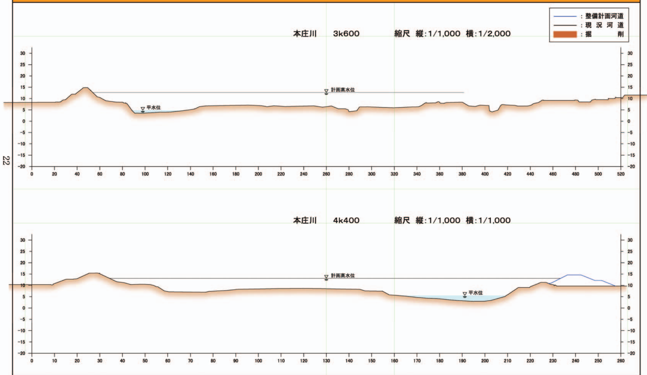
附図22 本庄川横断図(国土交通省)
