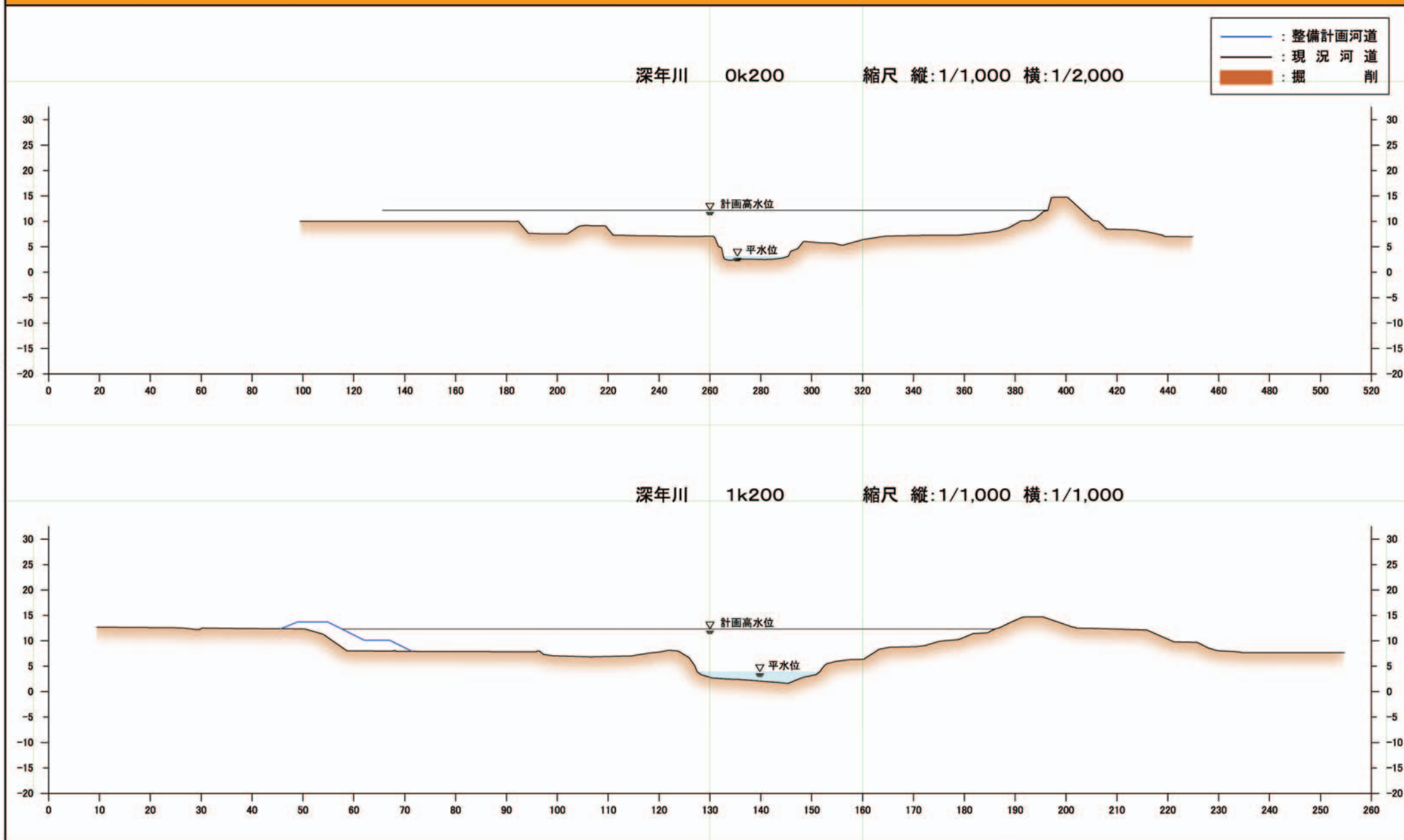
附図24 深年川横断図(国土交通省)
