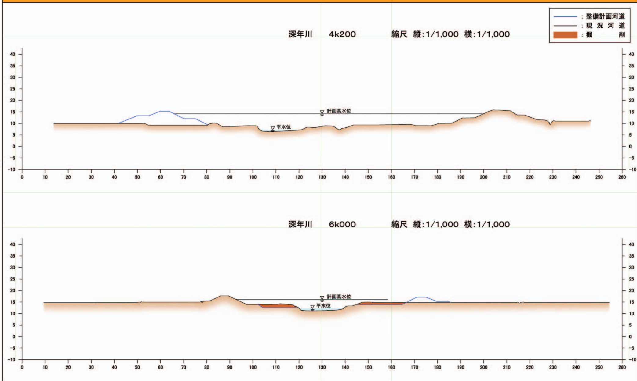
附図26 深年川横断図(国土交通省)
