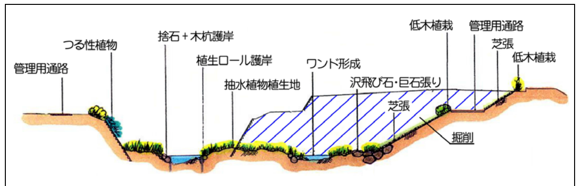
図 4.2.27 水流川の整備イメージ (宮崎市大塚町)
