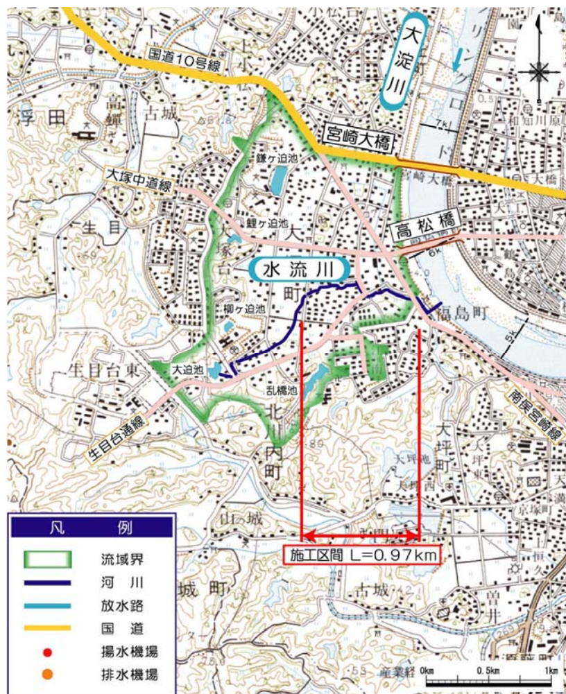
図 4.2.28 施工区間(水流川)
