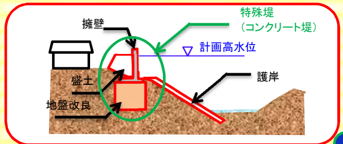
特殊堤断面イメージ図
