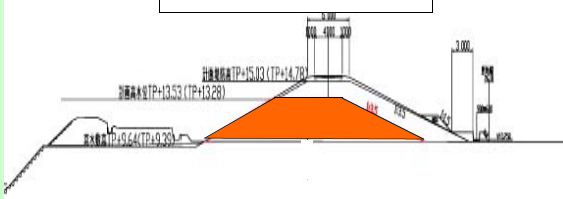
吉野地区暫定盛土断面図
