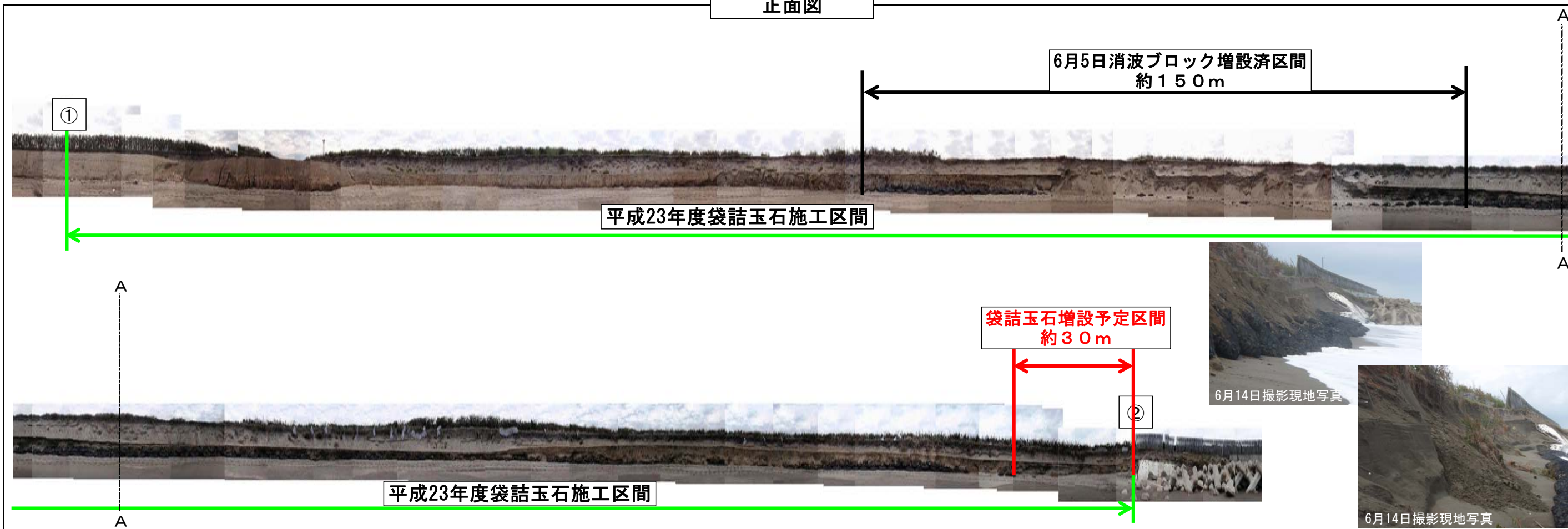
正面図
