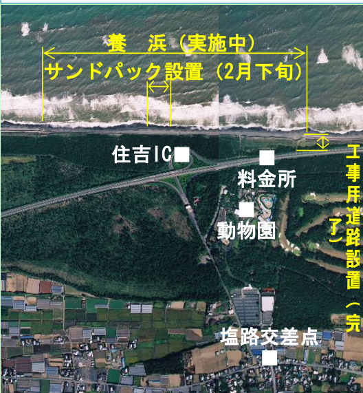
養浜実施中 (H24. 2. 16撮影)
