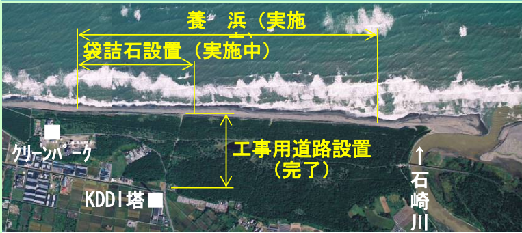
養浜・袋詰石実施中 (H24. 2. 10撮影)
