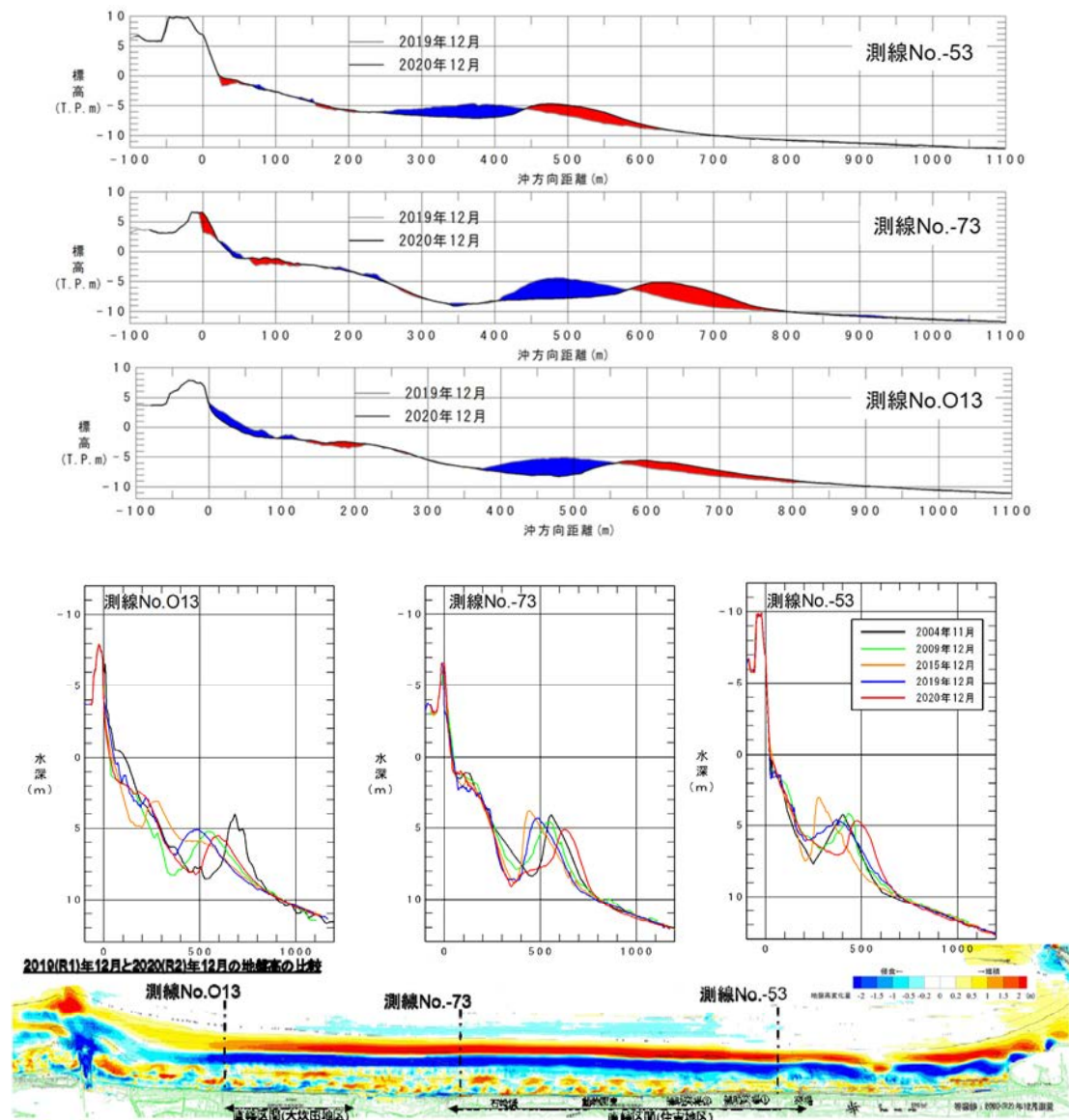
図ー 3.9 2019 (R1) 年から 2020 (R2) 年の横断変化図
