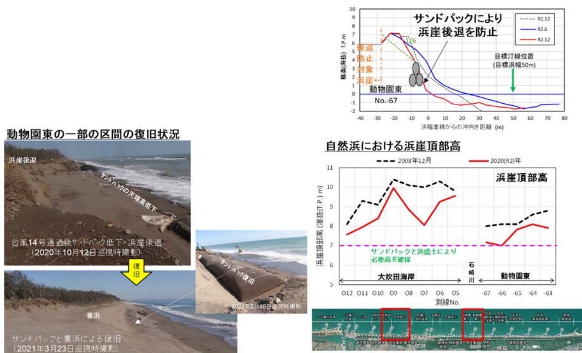
図－ 3.15 浜崖頂部高の変化および動物園東埋設護岸設置区間の浜崖形状の変化
