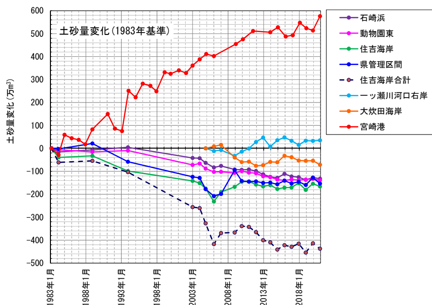
図－ 3.5 宮崎海岸周辺の土砂量変化
