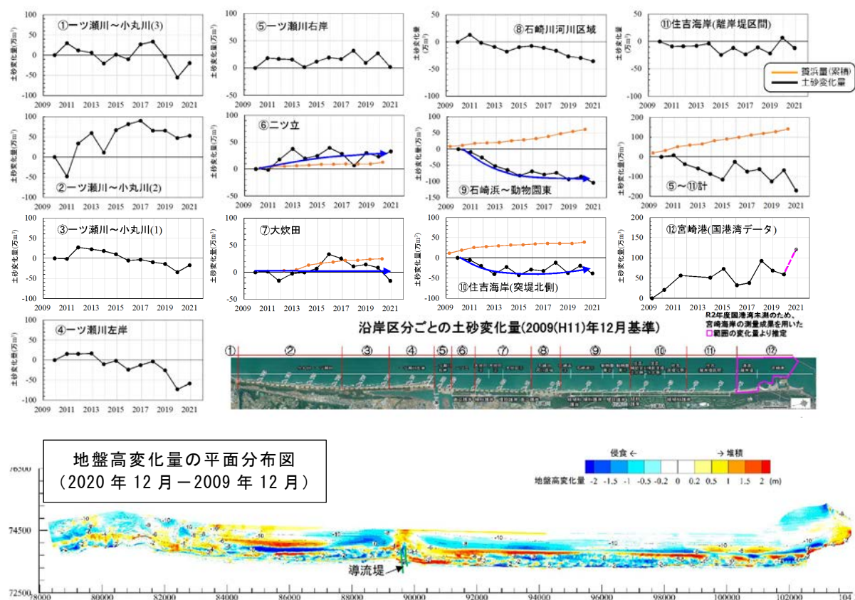
図－ 3.7 沿岸区分毎の土砂変化量 (2009 (H21) 年 12 月基準)
