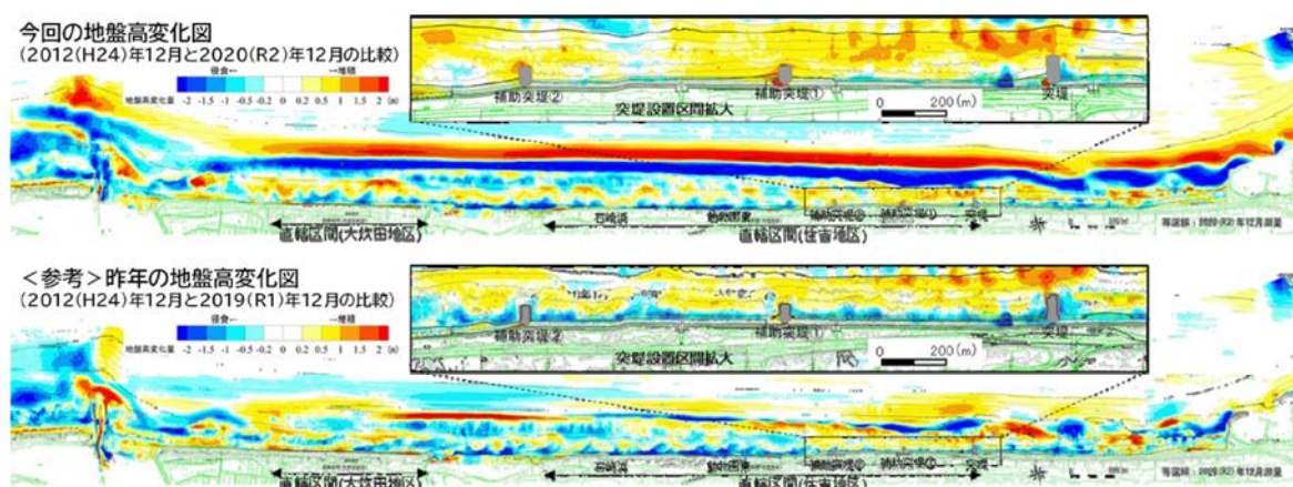
図－ 3.8 地盤高変化量の平面分布
