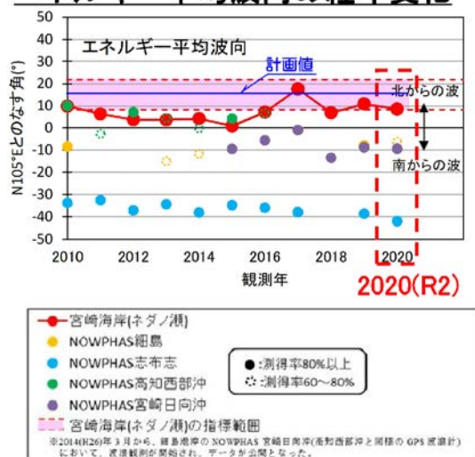
図ー 3.4 宮崎海岸および近隣のエネルギー平均波向の経年変化
