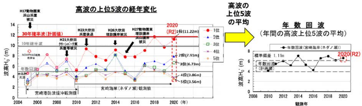
図－3.1 高波浪来襲状況
