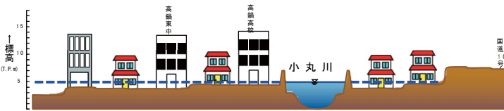
○小丸川堤内地横断面図（高鍋市街部）
