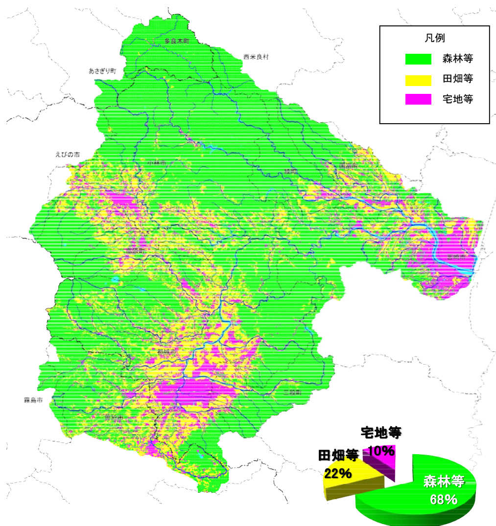
図 1.1.10 大淀川流域における土地利用図
