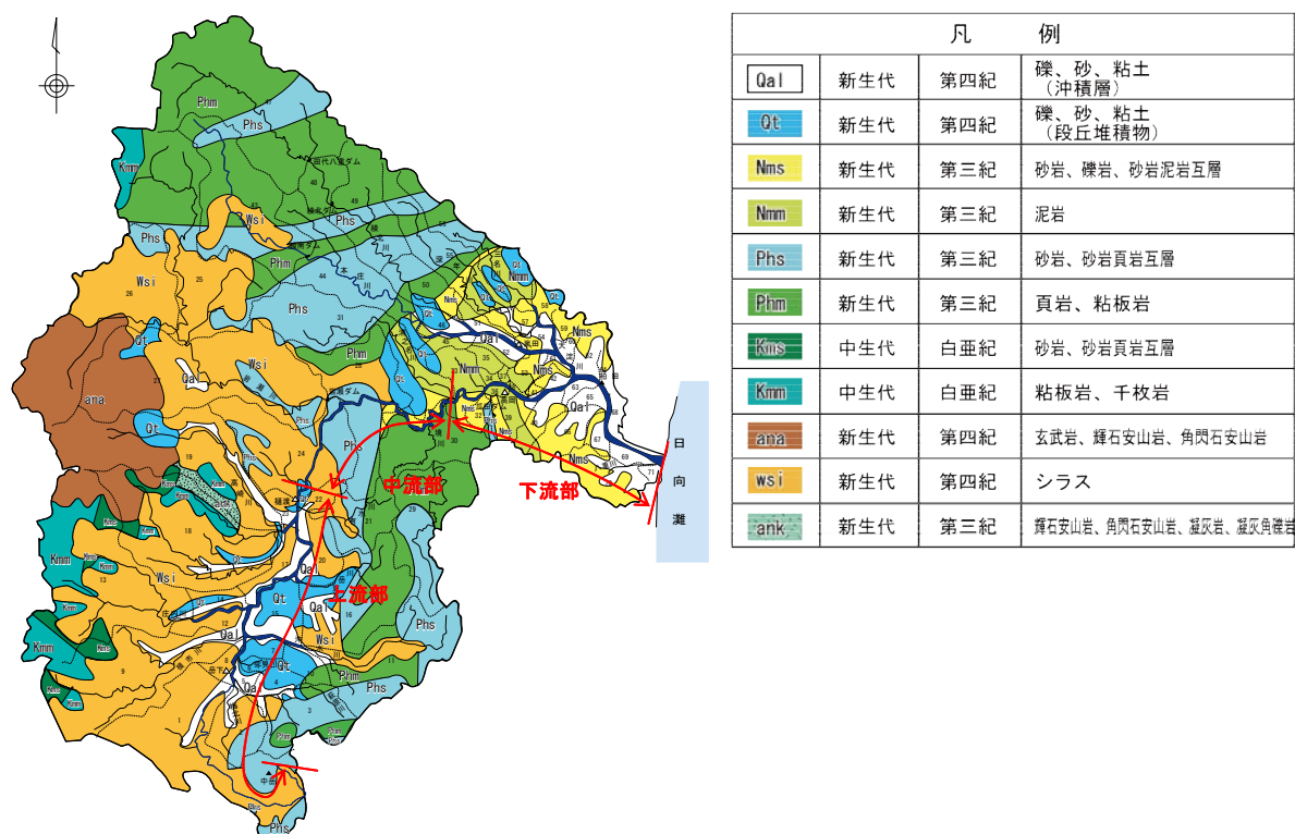
図 1.1.4 大淀川流域地質図
