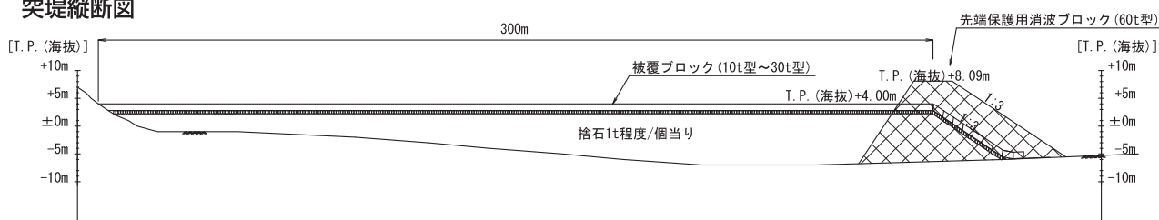
突堤縦断面図
