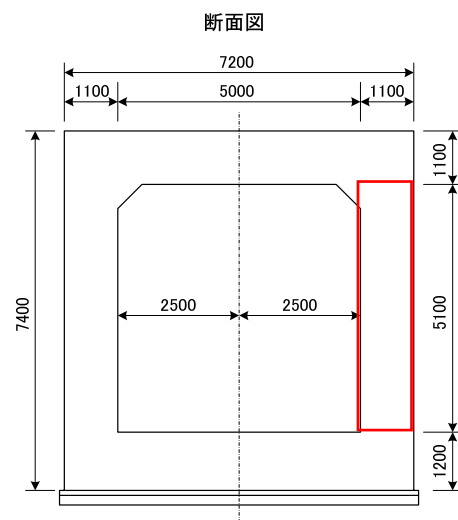
図 4.6.1 算出範囲
