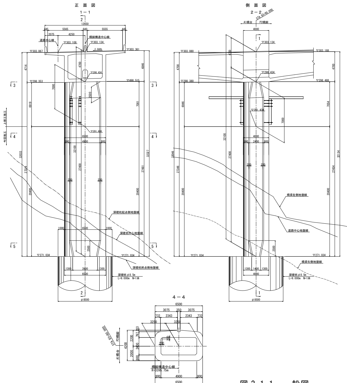
図 3.1.1 一般図
