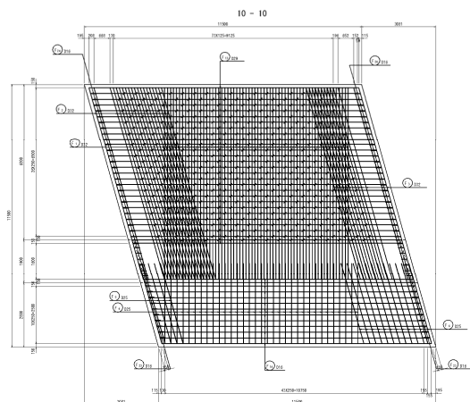
前フーチング詳細図 S=1/20
