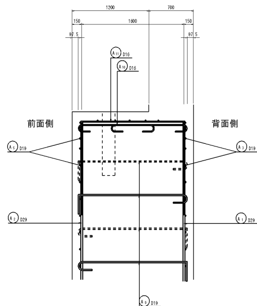
縦壁詳細図
