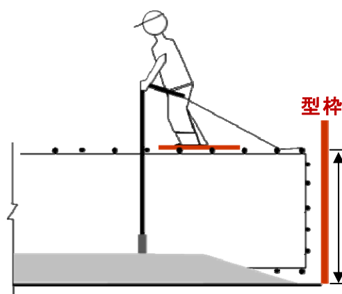
図 1.6.2 締固め作業高さ
