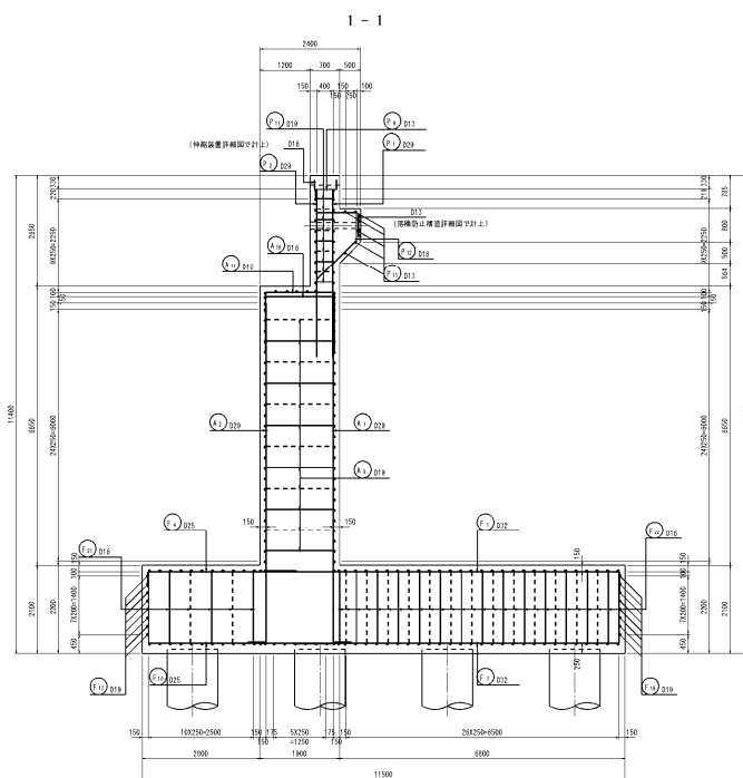
図 2.1.3 一般配筋図
