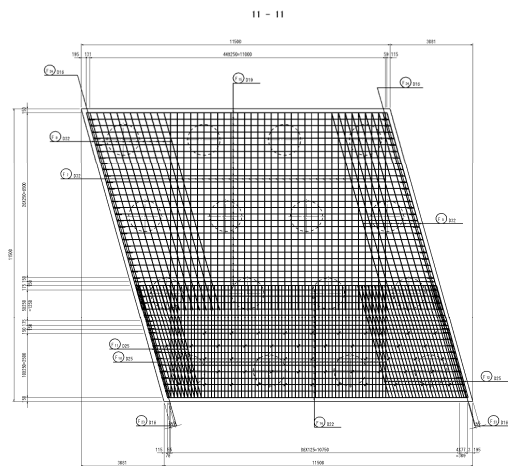
後フーチング詳細図 S=1/20
