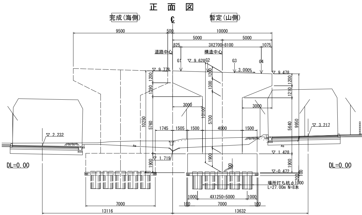
图 1.1.1 下部工一般图
