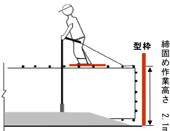
図 2.2.2 締固め作業高さ
