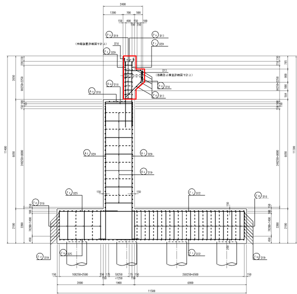
図 2.2.5 算出範囲
