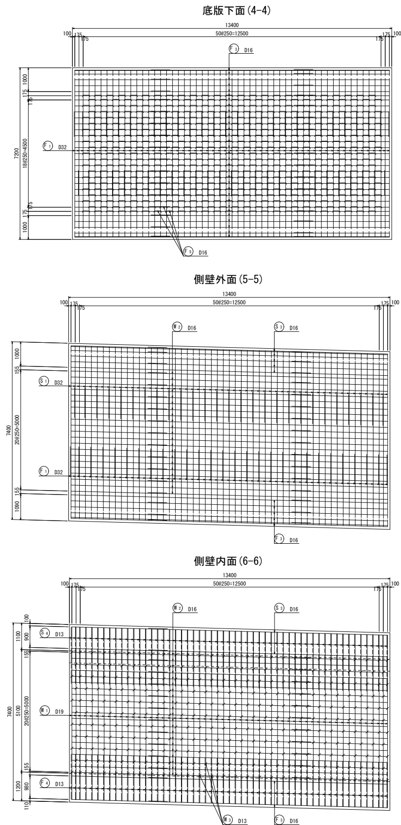
図 4.1.3 ボックスカルバート配筋図 (その 2)
