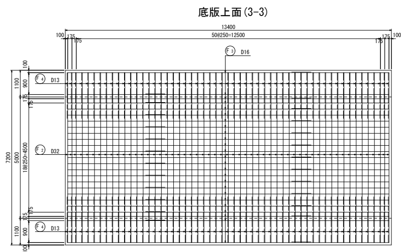
図 4.1.2 ボックスカルバート配筋図 (その 1)
