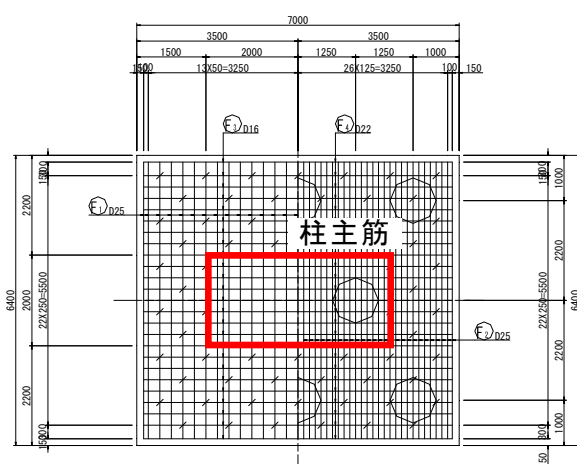
图 1.6.1 柱主筋位置
