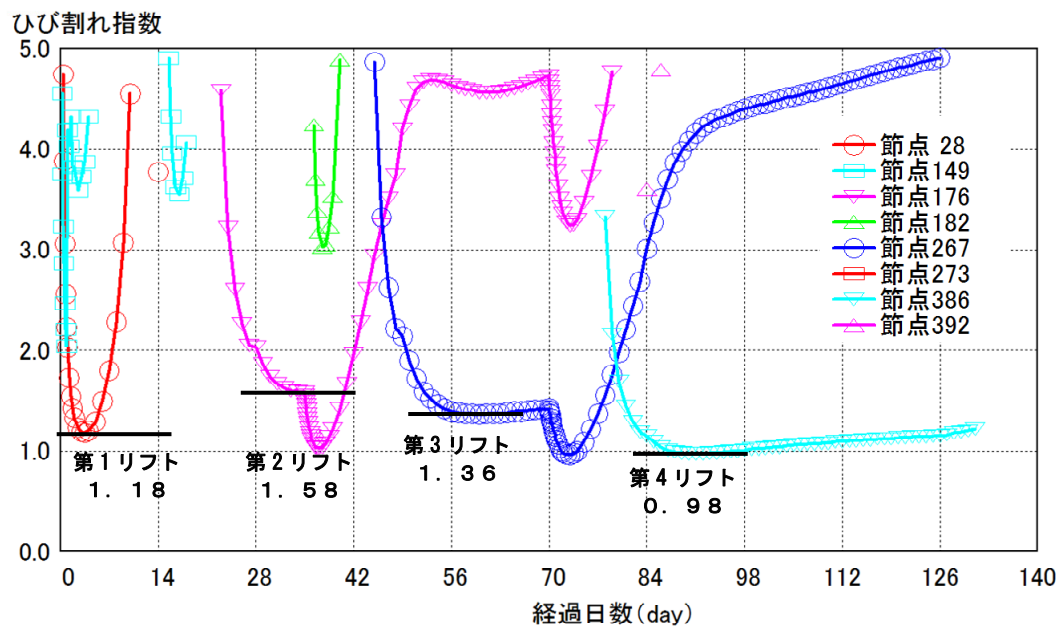
図 1. 7. 10 材齢とひび割れ指数の関係（対策パターン）
