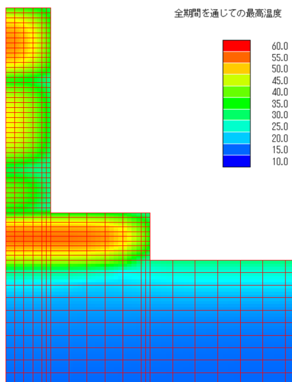
図 1.7.9 最高温度分布図（対策パターン）
