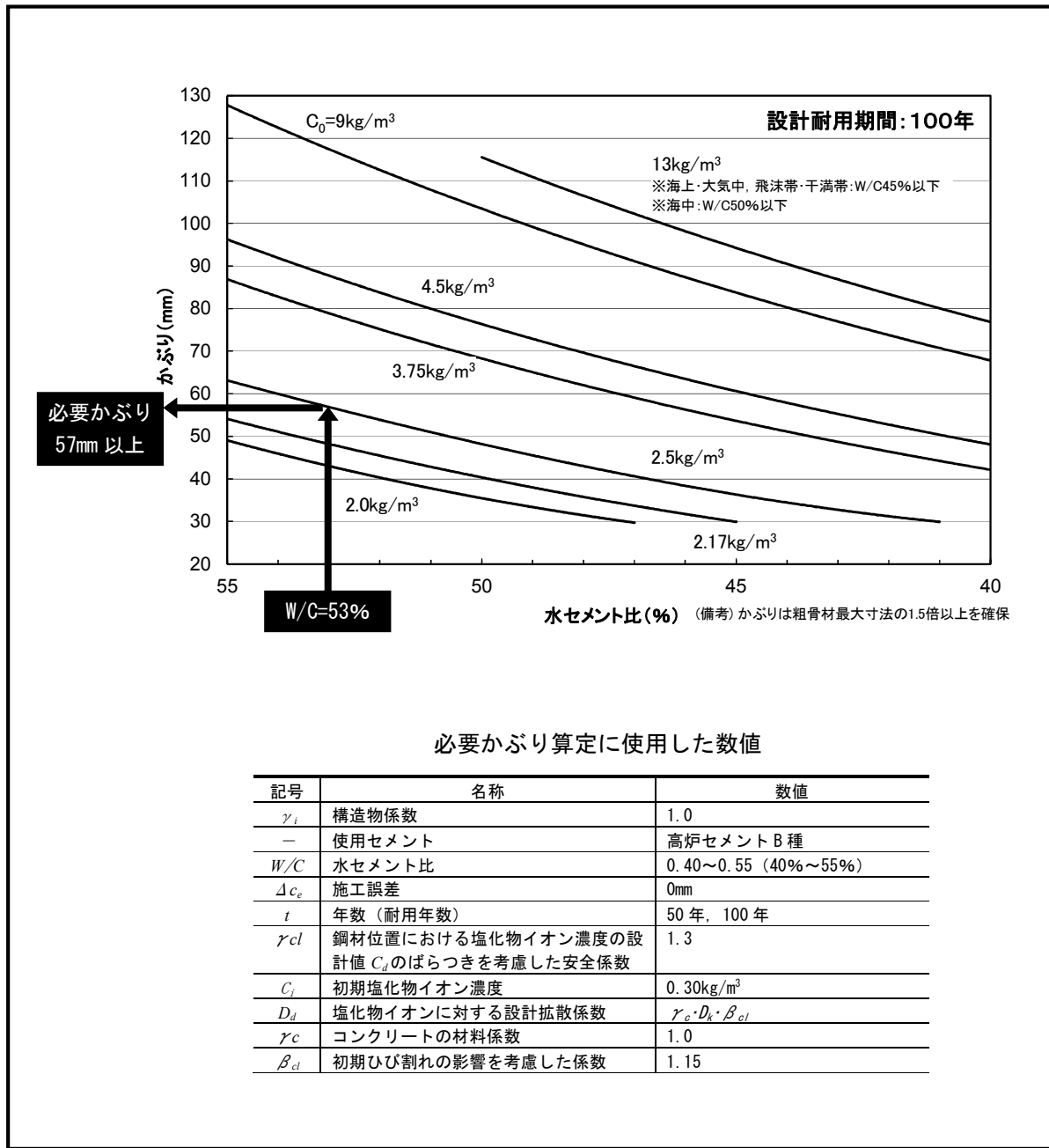
図 1.3 塩害に対する照査を満足する水セメント比およびかぶり判定図
