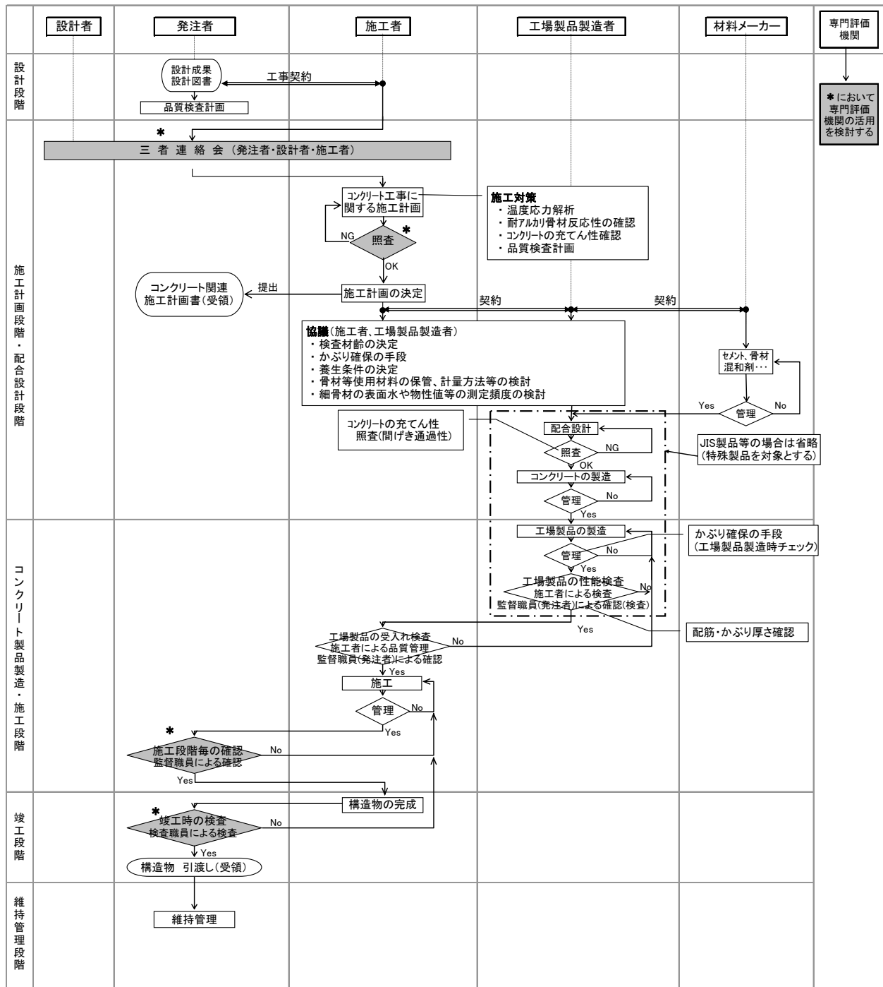
解説 図 1.2.4 施工計画段階以降における建設プロセス （その2：工場製品使用）
