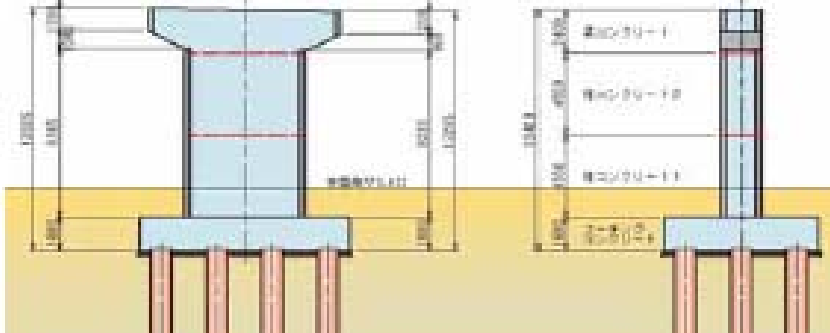
図 2-2 P2 橋脚コンクリート割付図
