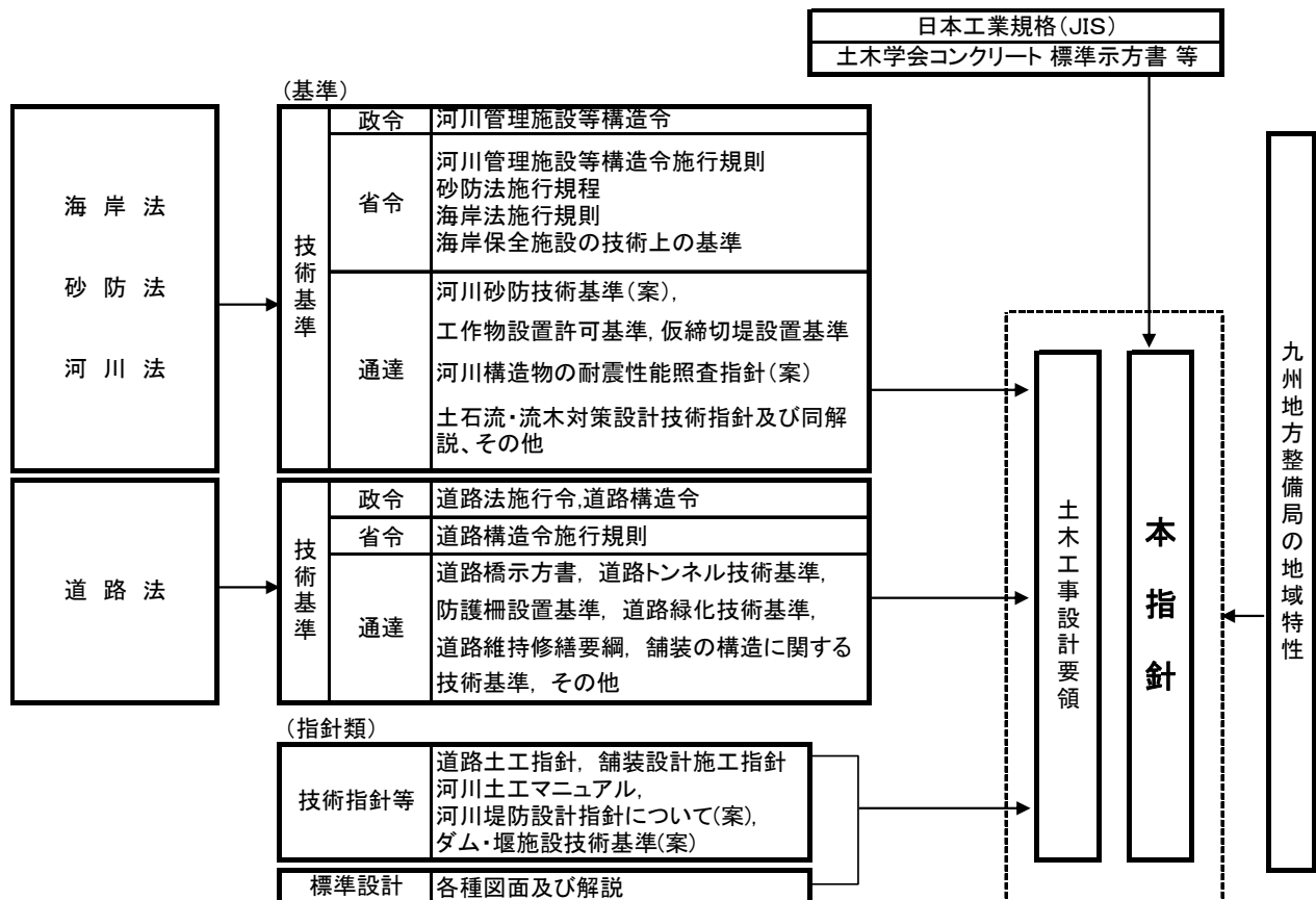
解説 図 1.1.3 各種基準類および本指針の位置づけ
