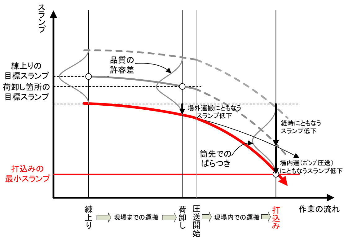
解説 図 3.1.2 スランプの経時変化の考え方
