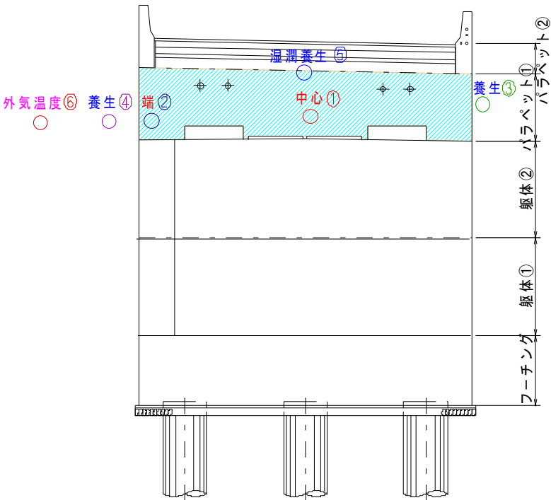
図 4-4 パラペット①計測位置
