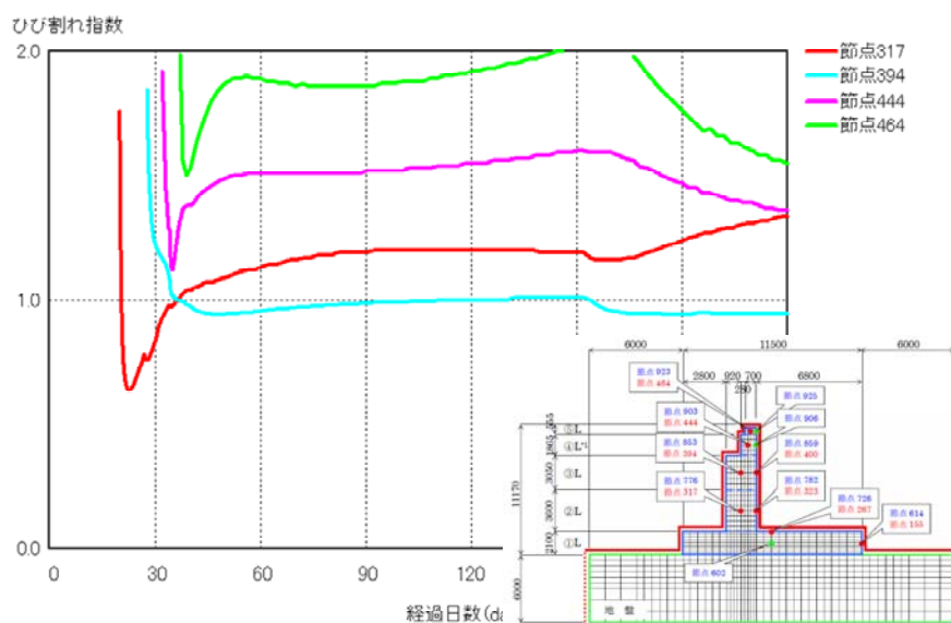
図 3-7 外部拘束によるひび割れ指数の経時変化（基本条件）
