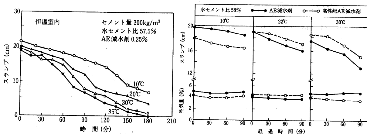
解説 図 3.13.1 コンクリートのスランプの経時変化（温度別）
