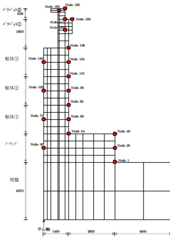
図 3-2 解析モデル図 Case2, 4, 5, 6, 7, 8
