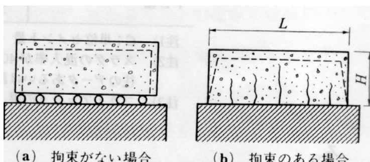
ii) 外部拘束によるひび割れ（壁状構造物）
