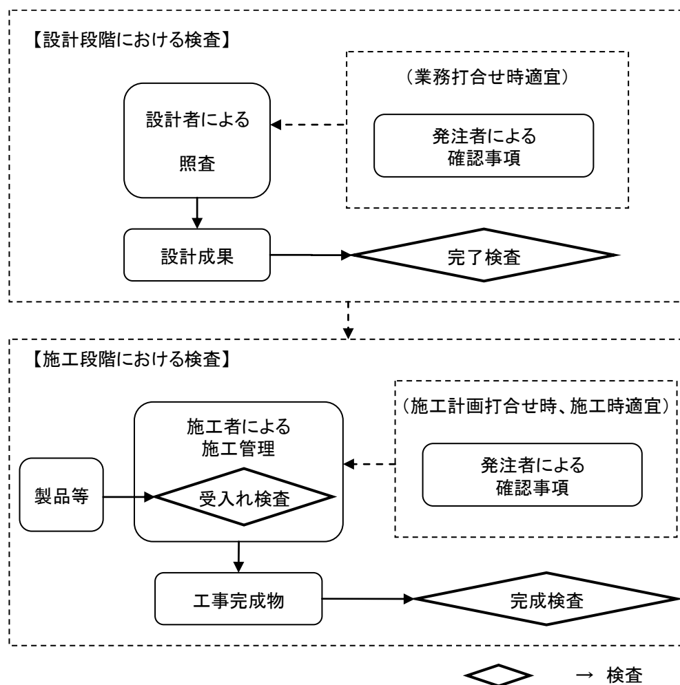
解説 図 7.1.1 本指針における検査の体系図
