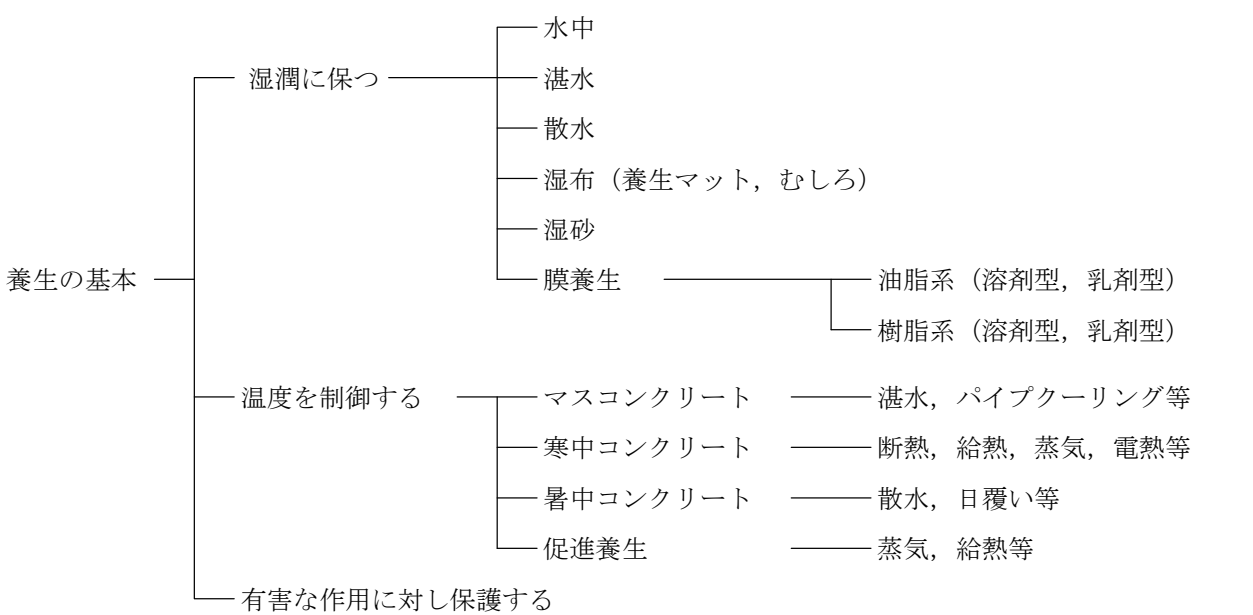
解説 図 3.8.1 養生の基本
