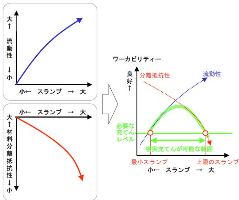
解説 図 3.1.1 密実充てんを達成するコンクリートのワーカビリティー
