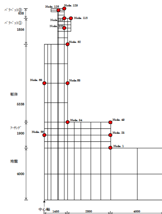
図 2-2 解析モデル
