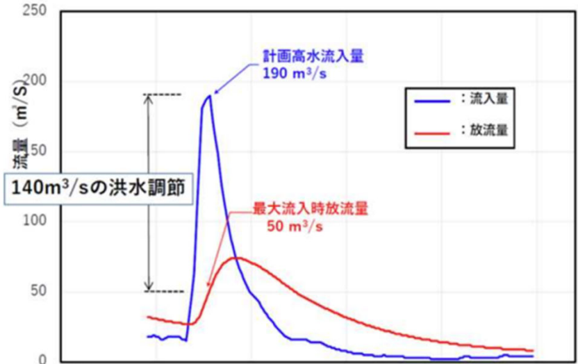
図2-2 小石原川ダム洪水調節計画図
