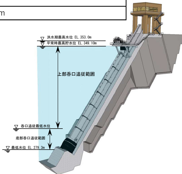
図5-24 選択取水設備模式図
