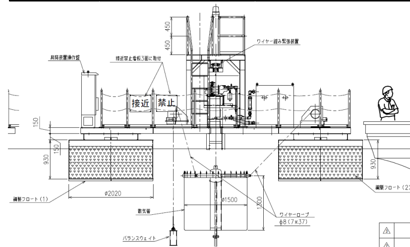
図5-25 曝気循環設備模式図
