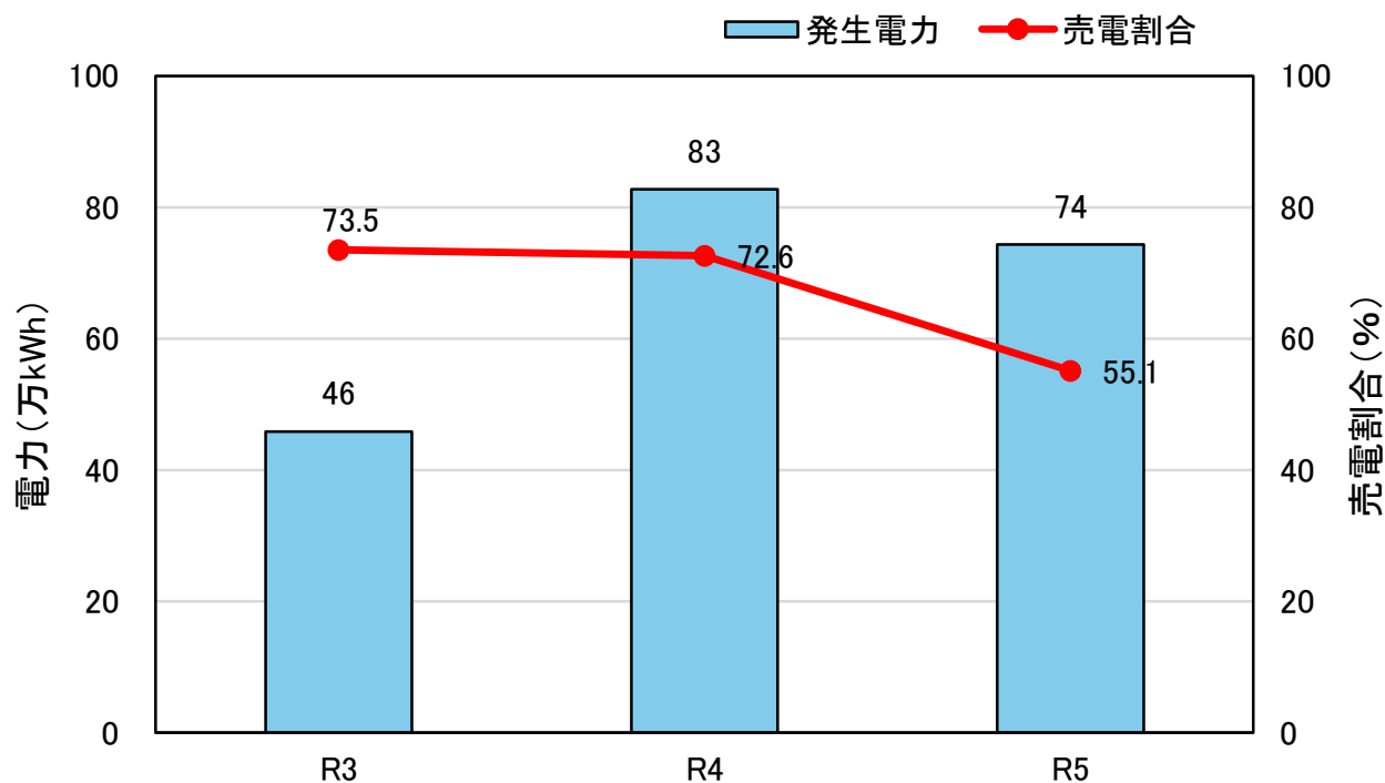
図3-8 発電実績
