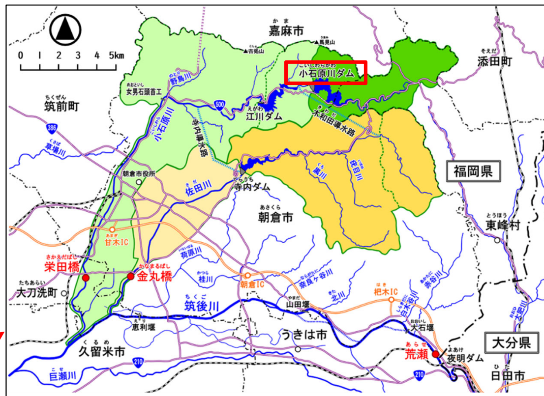
図1-1 全体位置図
