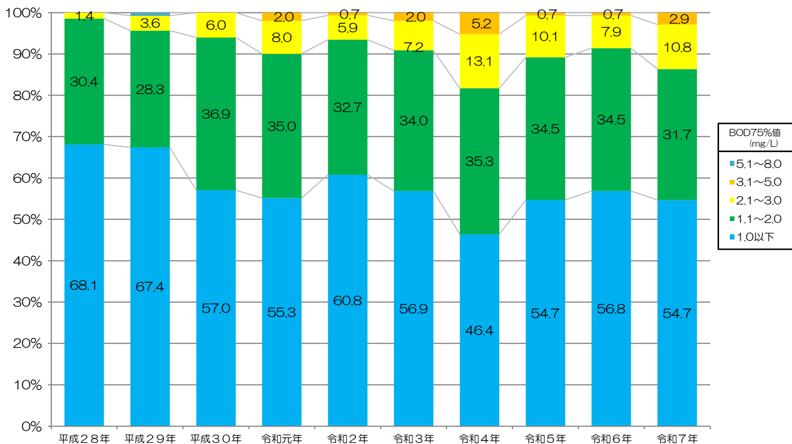
BOD75%値のランク別割合（平成28年～令和7年）
