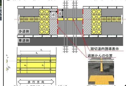
踏切内誘導表示の構造
