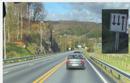
2+1車線（E39 ノルウェー）
