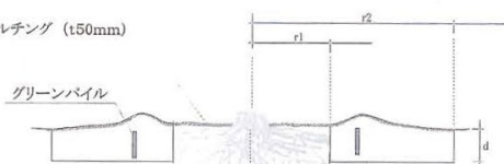
標準仕様図 (2) ~ (6)
