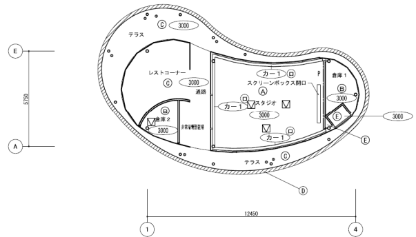
休憩施設 天井伏図
