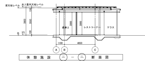
休憩施設 ニーニ 断面図
