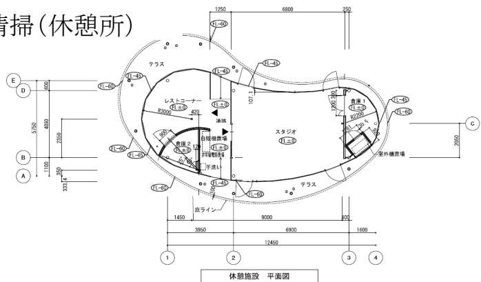
休憩施設 平面図
