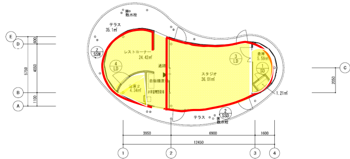
休憩施設 建具符号
