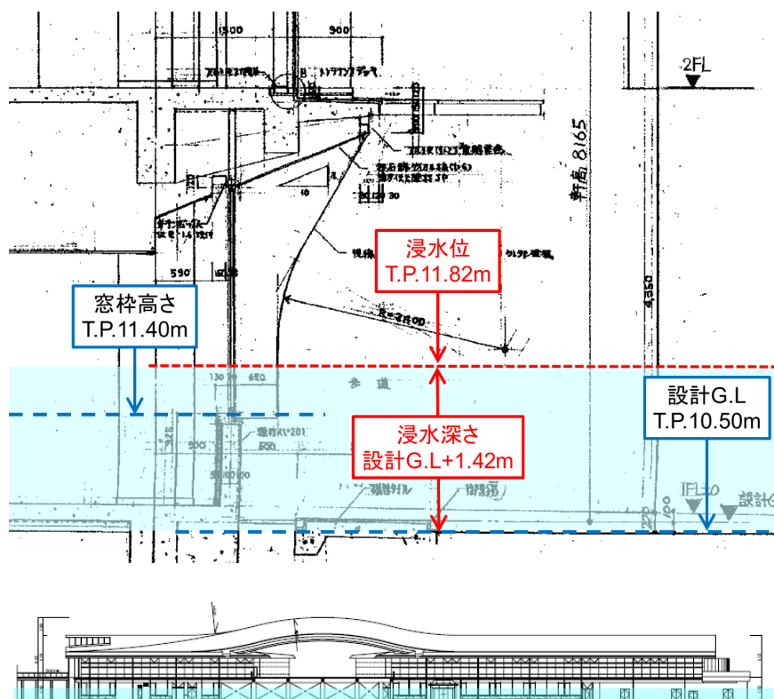
歴史公園センター各部の高さ
