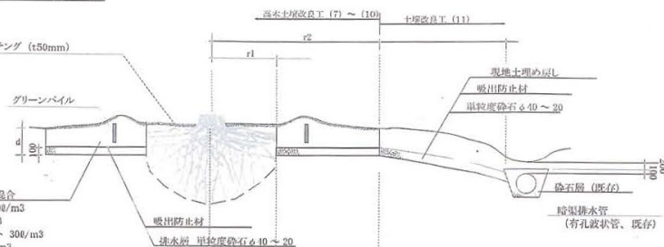
標準仕様図 (7) ~ (10)、(11)
