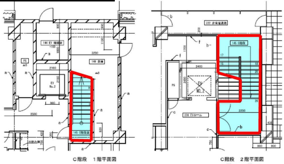
145 定期清掃 床清掃1（階段詳細）
