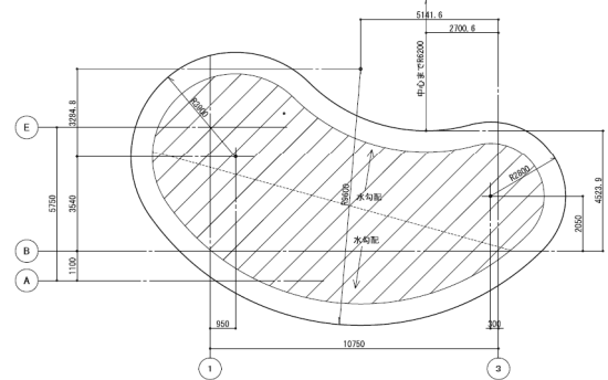
休憩施設 屋根伏図
