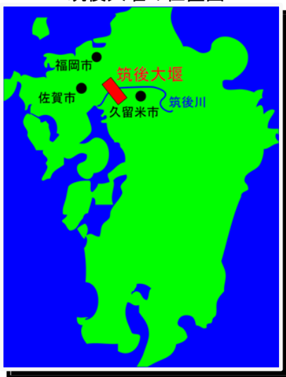
筑後大堰の位置図
